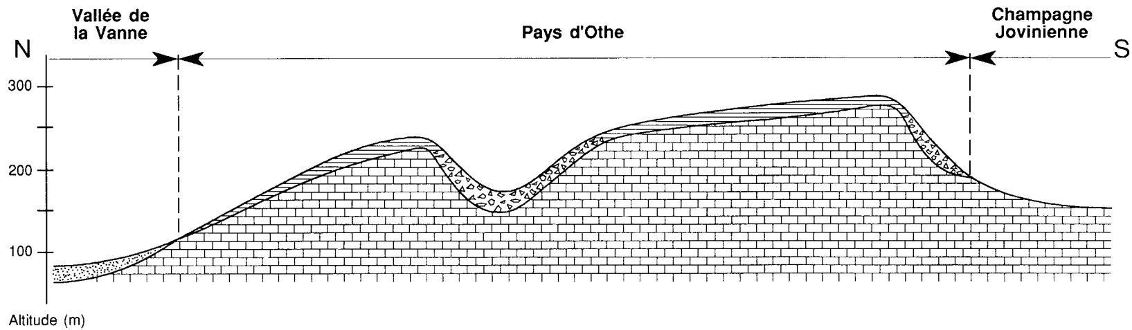
Figure 1 : Coupe géologique simplifiée du Pays d'Othe.
