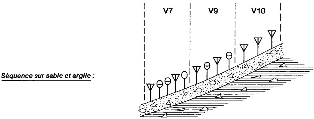
Figure 7 : Schéma des relations matériaux-topographie-végétation des stations forestières des versants.
