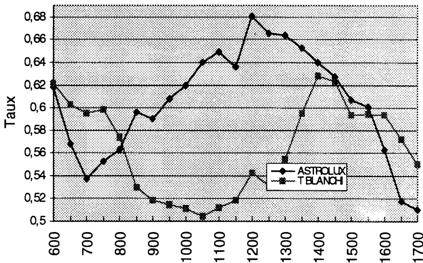
figure N°4 Taux moyens de transmission horaire du rayonnement global entre le 21/07 et le 18/08
