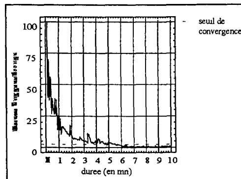
Figure 2 : courbe d'apprentissage.
