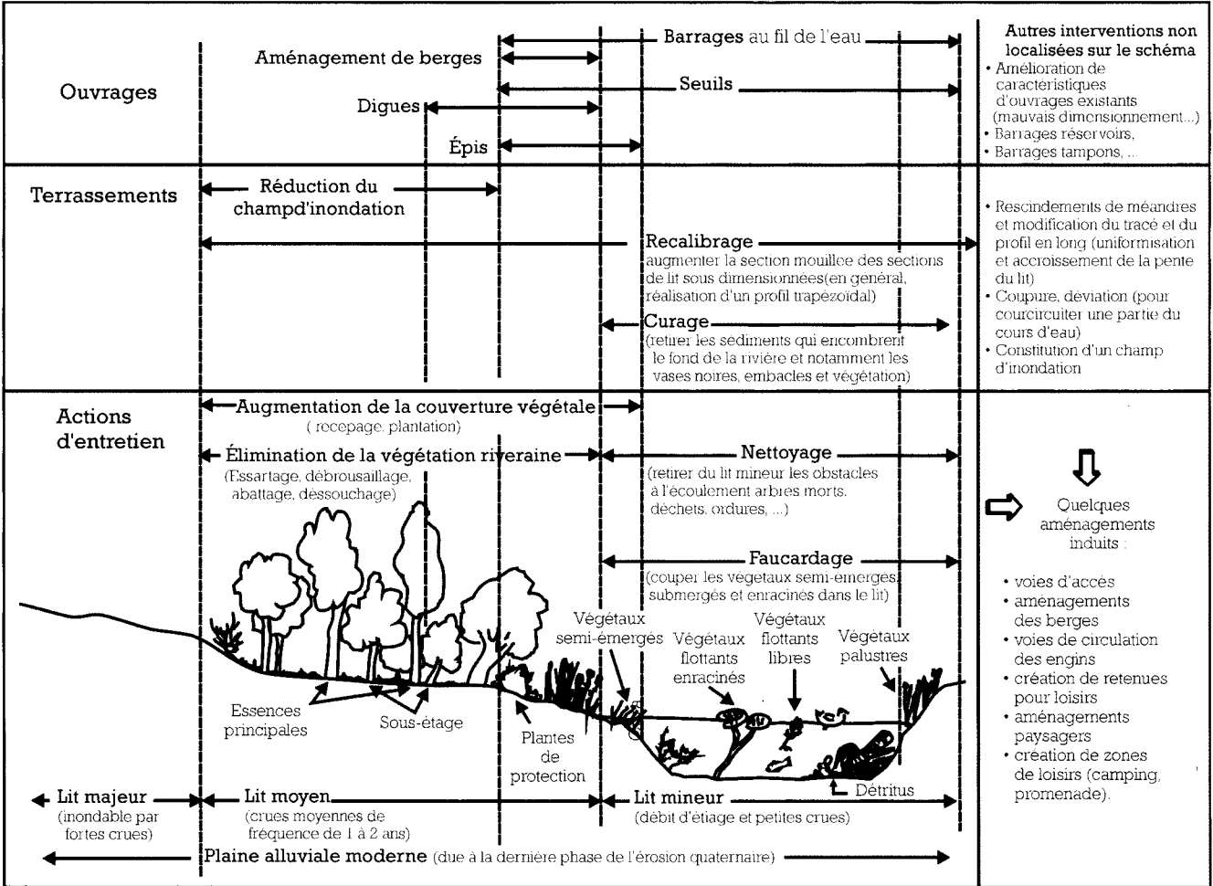
Figure 3.3 : La localisation des interventions sur une section complète de cours d'eau (Cemagref, 1983).
