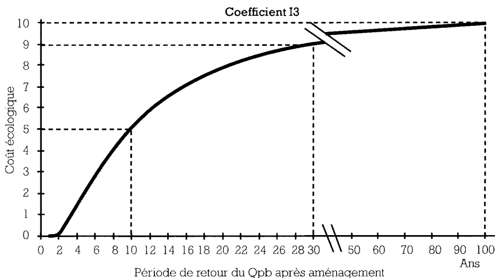
Figure 8.5 : Coût écologique de la réduction de la fréquence de débordement due à la chenalisation. La période de retour normale du débit de plein bord est généralement inférieure à 2 ans.
