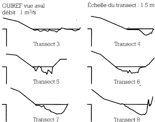
Figure 4.5 : Profil en travers de la station de référence du Guiers Vif.
