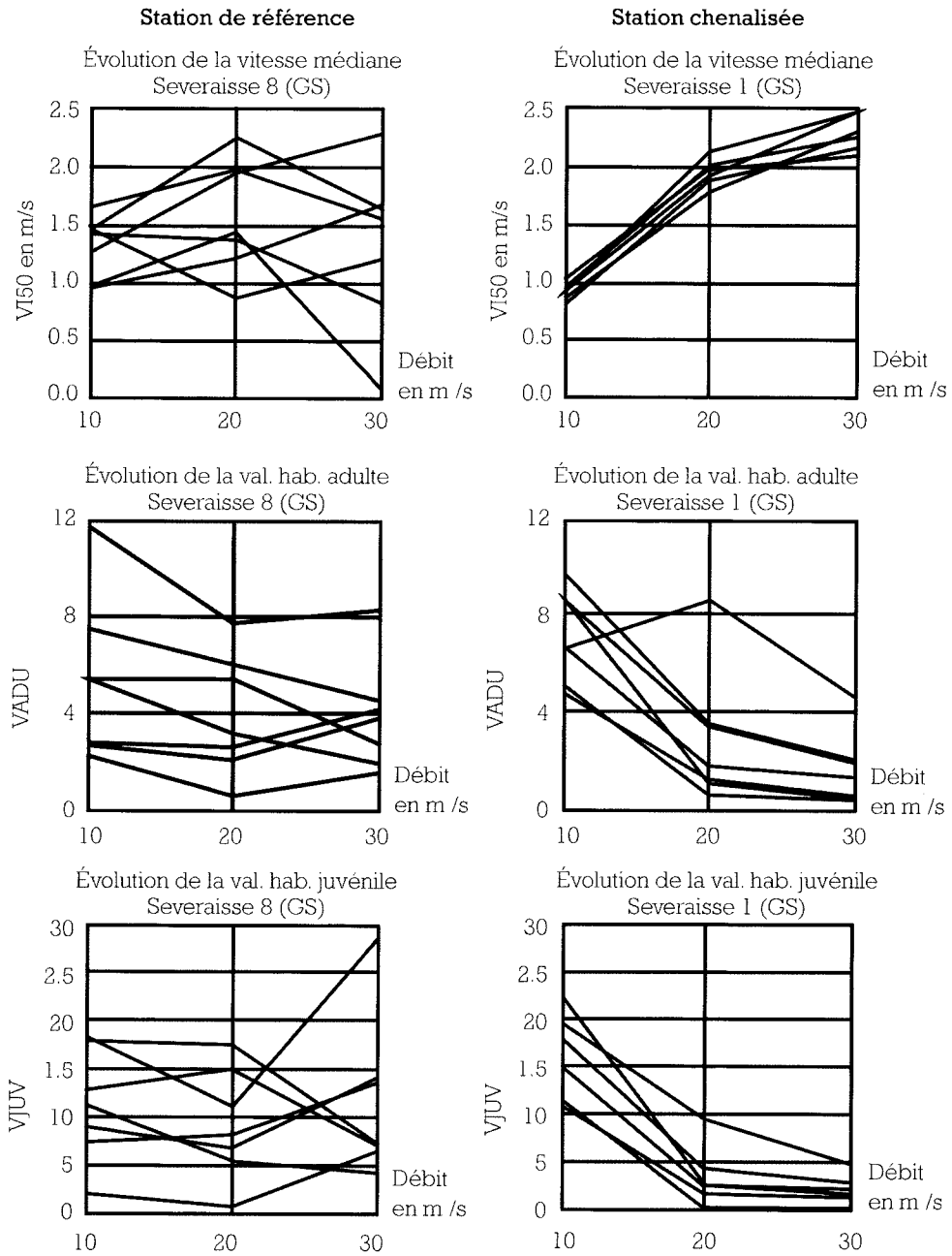
Figure 7.10 : La Severaisse (Hautes Alpes) : Profils d'évolution des vitesses médianes (VI50) et des valeurs d'habitat pour les adultes et juvéniles de truite fario en fonction du débit sur une station de référence (St. 8, AS) et sur une station chenalisée (St1, GS). D'après MALAVOI, 1990.
