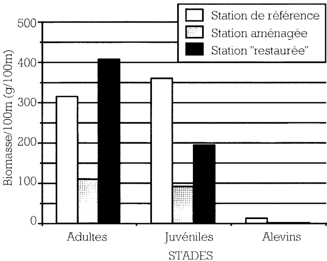
Figure 7.4 : Biomasses (rapportées à 100 mètres) des différents stades de truite ( Salmo trutta fario ) sur les trois stations du Guiers.
