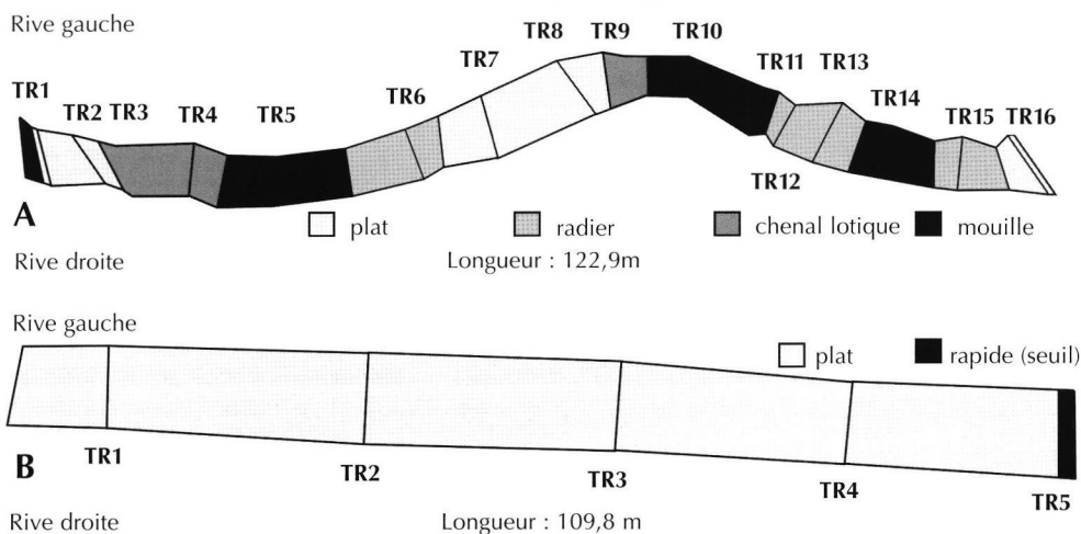
Figure 4.10 : Cartographie des faciès d'écoulement sur la station de référence (A) et la station aménagée (B) de l'Eau Morte.
