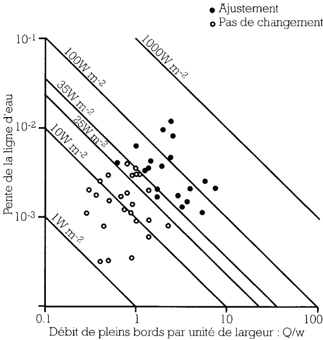
Figure 5.2 : Relation entre le débit de pleins bords par unité de largeur, la pente du lit et les ajustements observés au Royaume Uni suite à des interventions de type chenalisation (BROOKES, 1988).
