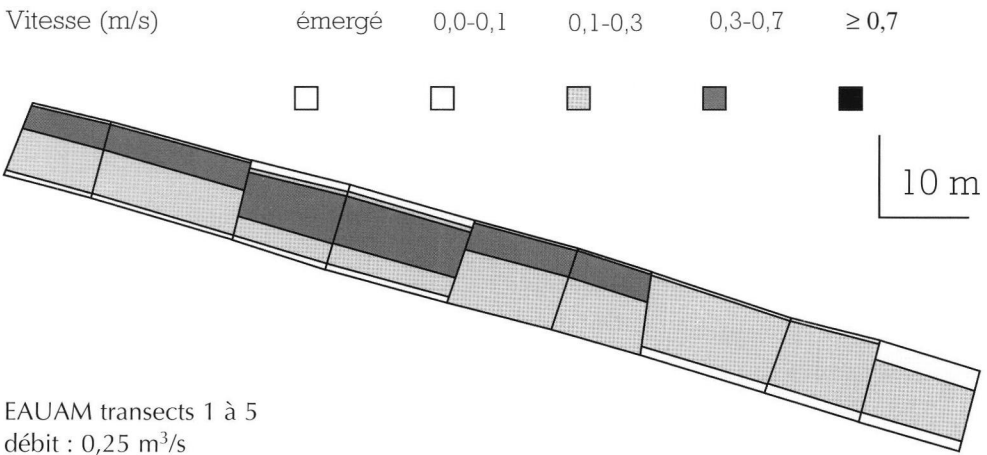
Figure 4.8 : Cartographie des vitesses sur la station de référence et la station aménagée de l'Eau Morte.
