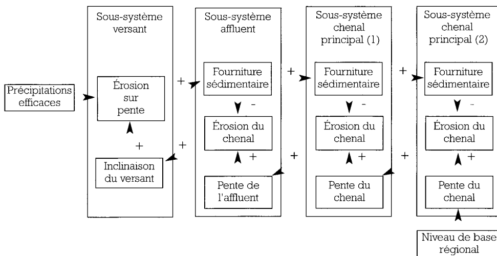
Figure 2.1 : Relation entre le chenal du cours d'eau et les systèmes du bassin ; un exemple de système géomorphologique simple est donné en A) montrant des relations positives (+) et négatives (-) entre la pente du tronçon ( i ), la taille des sédiments (le 50e percentile) du lit du cours d'eau ( D_{50} ) et la forme du profil en travers exprimé sous la forme du rapport profondeur ( p ) sur la largeur ( l ). B) montre le système comme élément d'un système à processus-réponse dans lequel les variables morphologiques sont ajustées aux changements de débits ( Q_L ) et de charge sédimentaire ( Q_s ). En C) des boucles de rétroaction négative connectent des systèmes en cascades et des systèmes géomorphologiques ; elles illustrent la séquence complexe d'interactions entre les secteurs du chenal principal, les affluents et les versants, résultant d'un changement des précipitations efficaces ou du niveau de base régional. Les changements induits dans la morphologie du chenal ( i , D_{50} , p/l ) pouvant être interprétés en référence à A). Reproduit d'après PETTS & BRAVARD (1993) avec autorisation.
