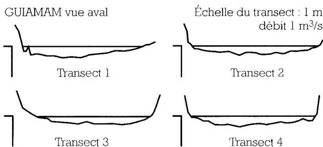
Figure 4.6 : Profil en travers de la station aménagée du Guiers Mort aval.
