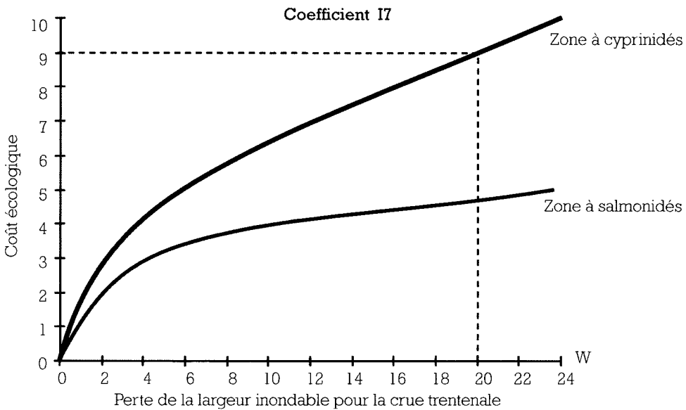
Figure 8.8 : Coût écologique de la perte de la connectivité latérale estimé par la perte de largeur inondable pour la crue trentennale.
