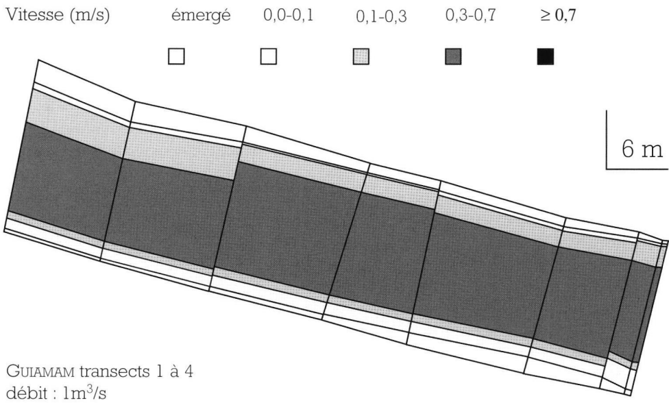
Figure 4.7 : Cartographie des vitesses sur le Guiers vif (station de référence) et sur le Guiers Mort aval (station aménagée).
