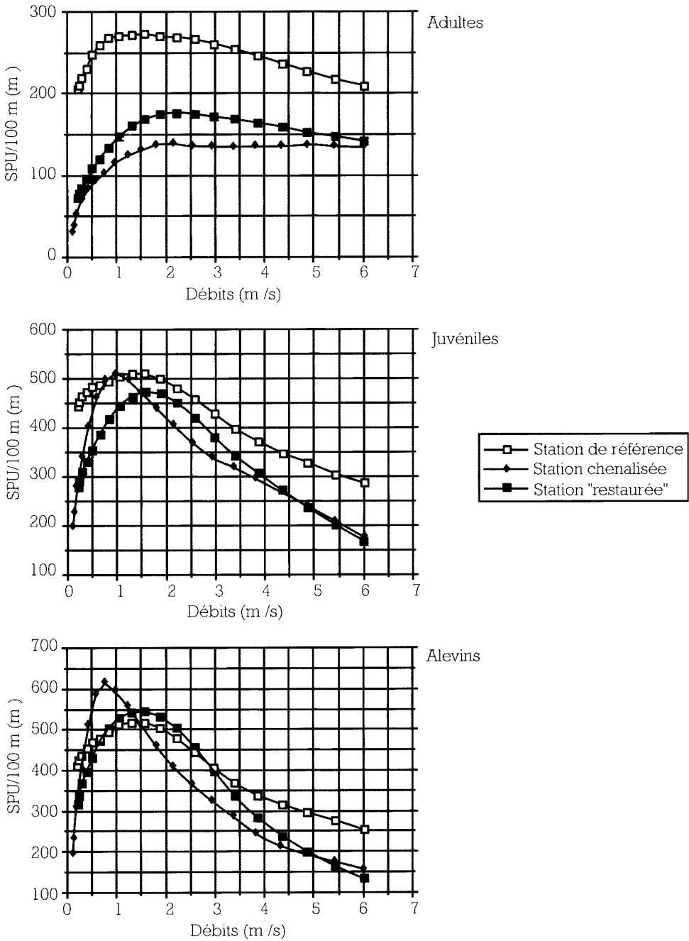
Figure 7.5 : Évolution avec le débit de la surface pondérée utile par 100m (SPU/100m) pour les différents stades de la truite ( Salmo trutta fario ) sur les trois stations du Guiers.
