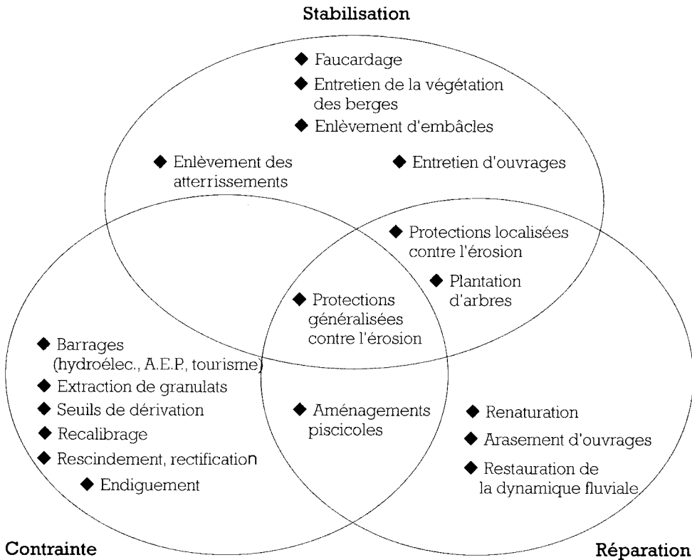
Figure 3.4 : Typologie des interventions humaines touchant le milieu physique d'eau courante (adaptée d'après Malavoi, 1990).
