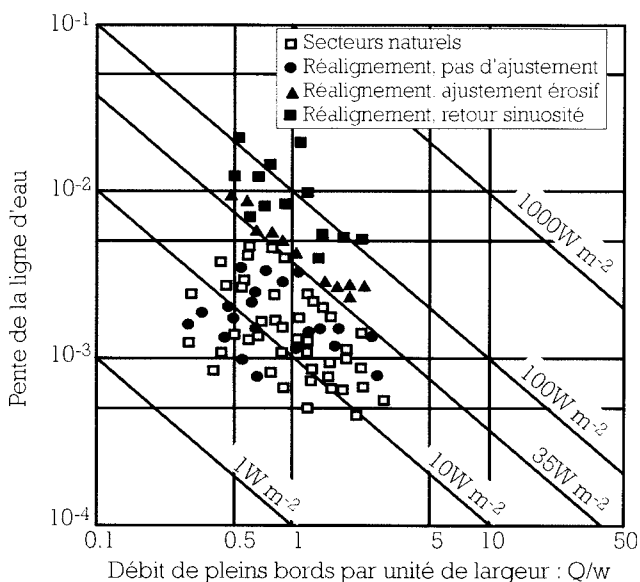
Figure 5.1 : Exemples de réajustements consécutifs à des travaux de rectification sur des cours d'eau danois. Chaque site est caractérisé par son débit de plein bord par unité de largeur et par la pente du lit (ce qui permet de tracer les droites d'énergie potentielle spécifique) (BROOKES, 1988).
