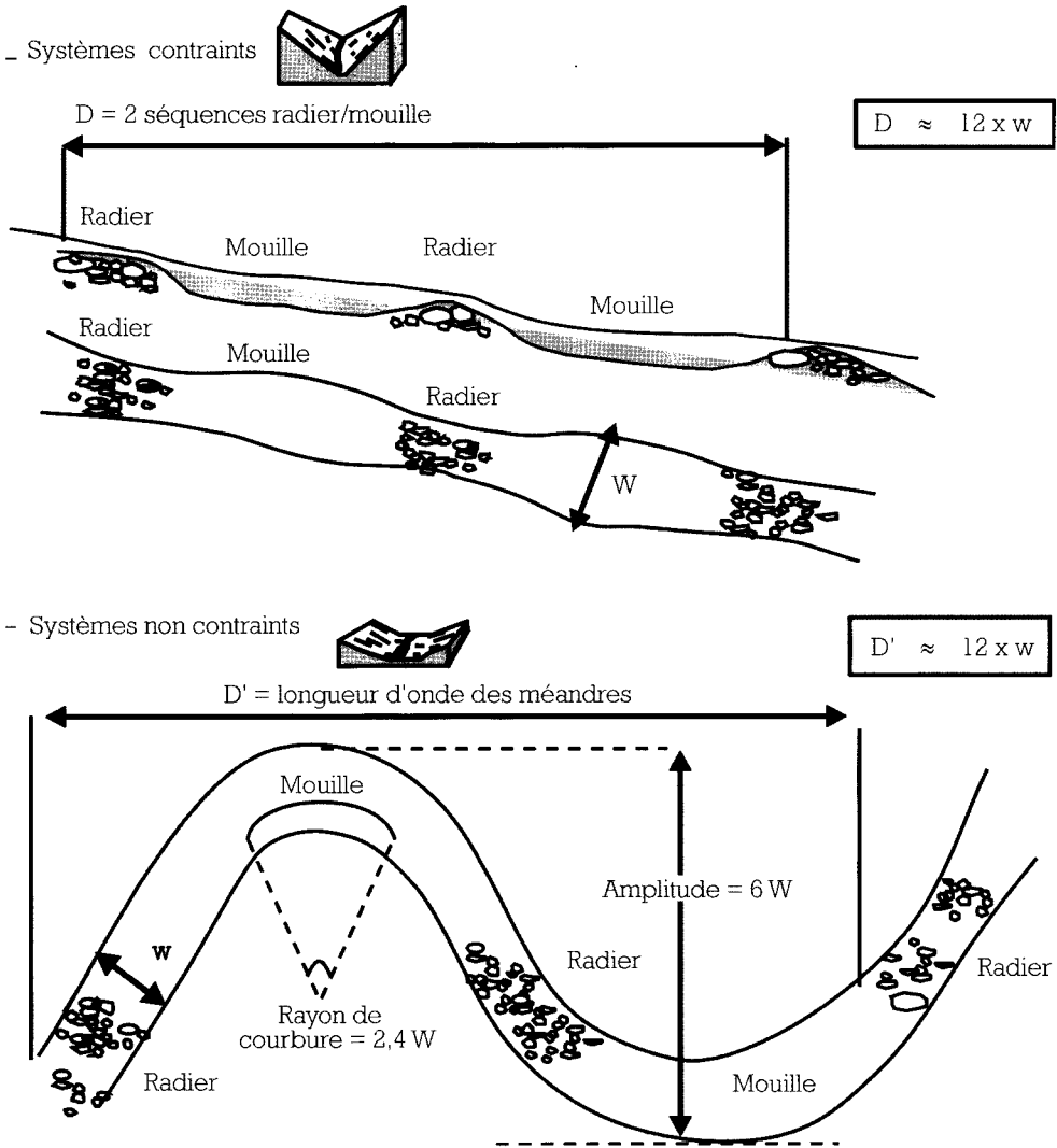
Figure 2.4 : Relation entre la géométrie du lit et la largeur au débit de plein bord ( W ).
