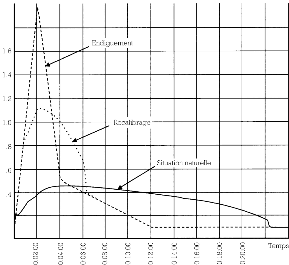
Figure 4.11 : Effets des aménagements sur les hydrogrammes de crue.
