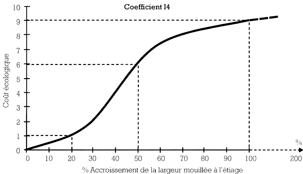
Figure 8.6 : Coût écologique de la chenalisation en fonction du pourcentage d'accroissement de la largeur mouillée à l'étiage.
