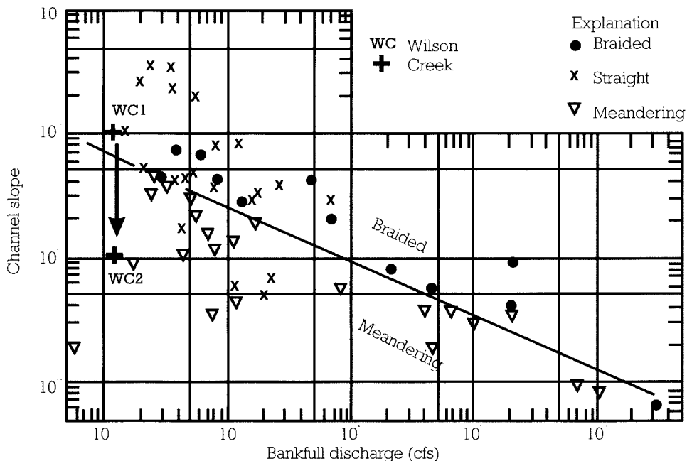
Figure 2.3 : Relations observées entre la pente (channel slope), le débit plein bord (bankfull discharge, en pied cubique/ seconde), et le type morphologique (braided : secteur en tresse, straight : rectiligne et meandering : à méandres) d'après LEOPOLD & WOLMAN (1957).
