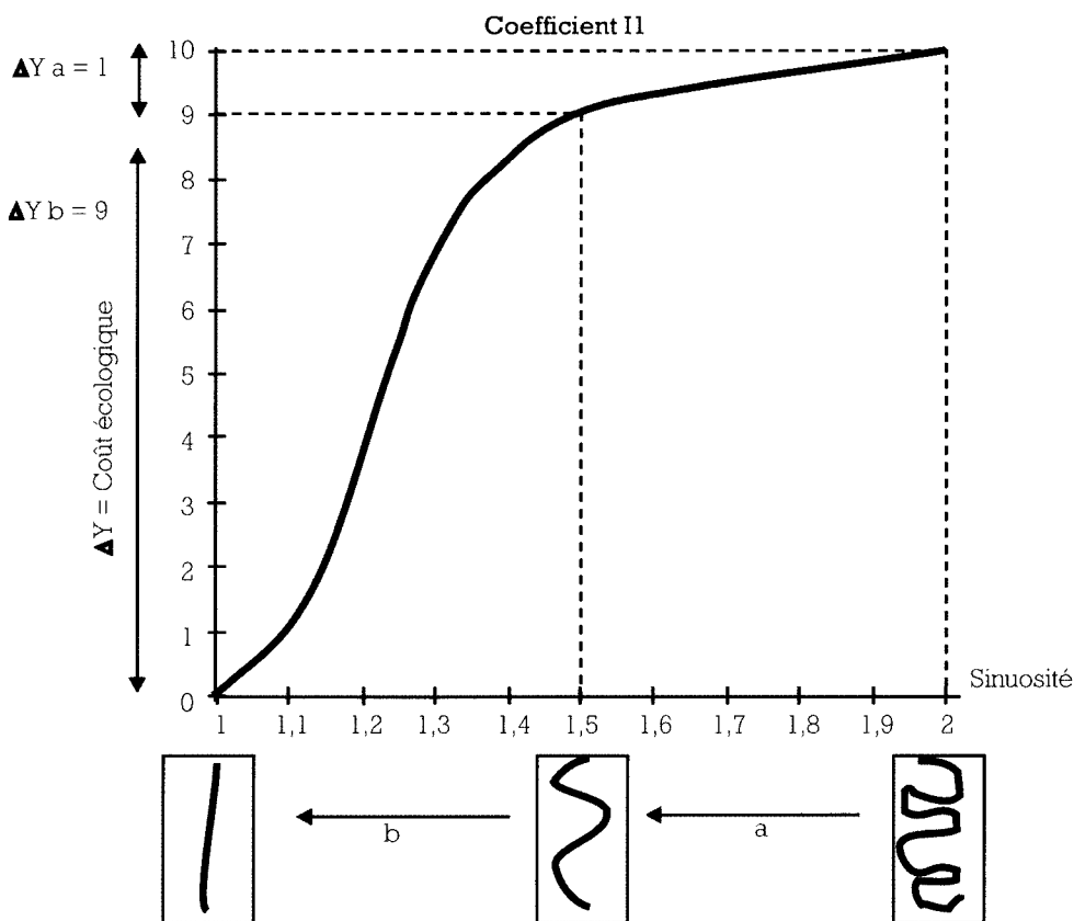
Figure 8.3 : Coût écologique de la perte de sinuosité par chenalisation. Le coût écologique se calcule par la différence ( \Delta y ) entre la sinuosité originelle du cours d'eau (état d'équilibre) et la sinuosité après aménagement.
