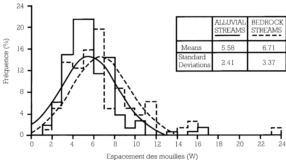
Figure 2.6 : Distribution de fréquence de l'espace des mouilles, mesuré en largeur plein bord ( W ) dans des cours d'eau alluviaux (trait plein) et des cours d'eau à fond rocheux (trait pointillé). Modifié d'après ROY & ABRAHAM (1980).
