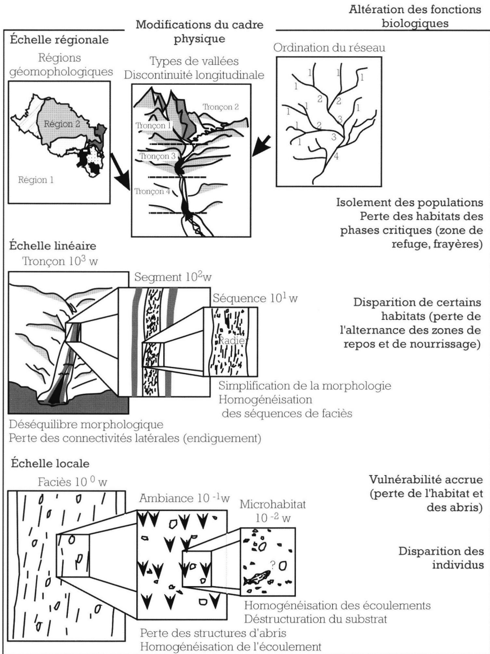
Figure 6.2 : Impacts de la chenalisation sur l'habitat et sur les fonctions biologiques aux différentes échelles physiques.
