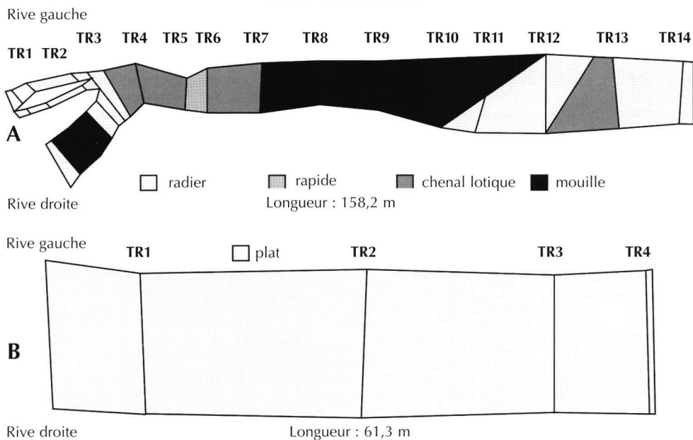
Figure 4.9 : Cartographie des faciès d'écoulement sur le Guiers vif (station de référence : A) et sur le Guiers Mort aval (station aménagée : B).
