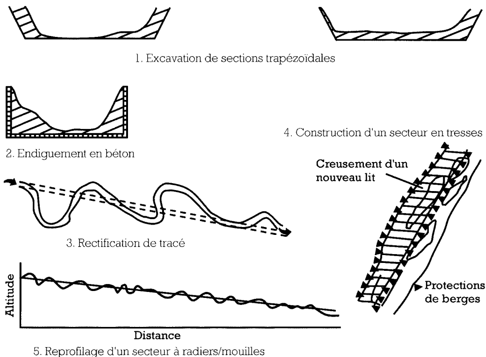
Figure 3.5 : Exemples d'aménagements en rivière (BROOKES, 1988).
