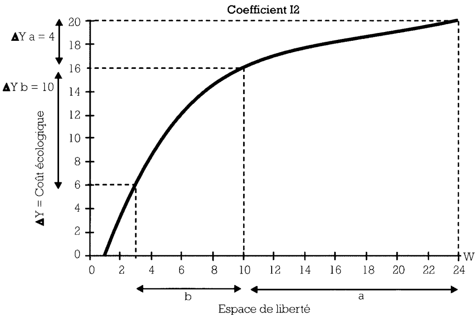
Figure 8.4 : Coût écologique de la réduction de l'espace de liberté due à la chenalisation. Le coût écologique se calcule par la différence ( \Delta Y ) entre la valeur de l'indice lue pour l'espace de liberté originelle et la valeur après aménagement.
