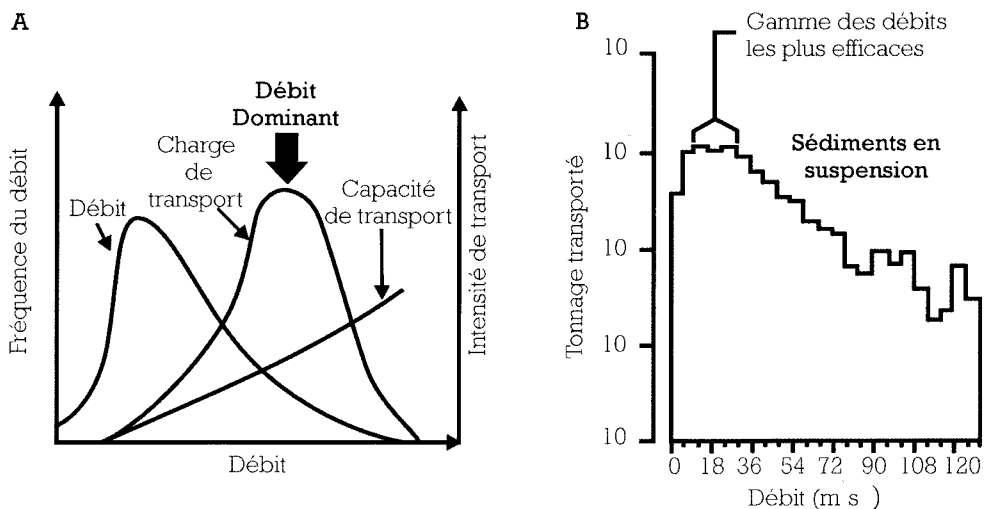
Figure 2.7 : A) Exemple de l'utilisation du débit dominant : la charge en sédiments totale transportée pour un débit donné est fonction de la fréquence de ce débit multipliée par la capacité de transport d'un débit de cette importance. Le débit dominant est celui pour lequel la charge est maximale ; B) débit dominant de la Wedy, Devon (WEBB & WALLING, 1982). Reproduit d'après GILVEAR & BRAVARD (1993) avec autorisation.
