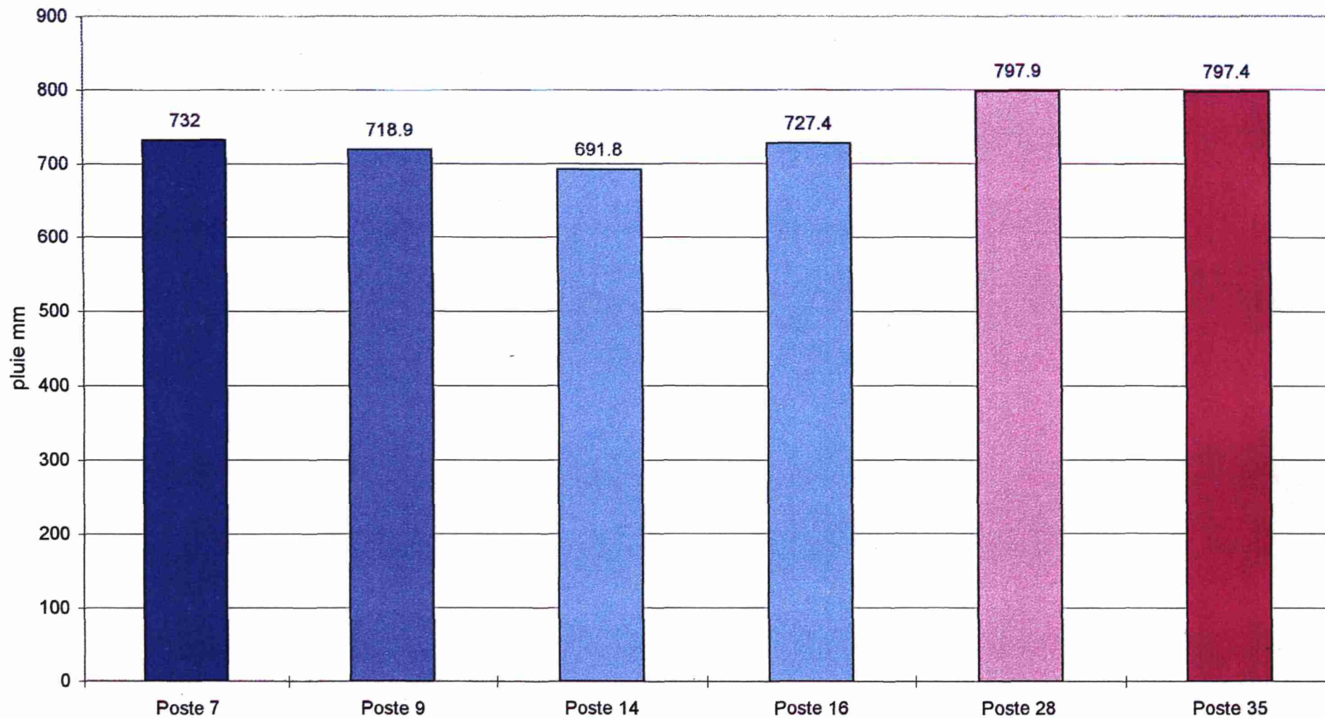
Comparaison des cumuls de pluie pour l'année 1998 suivant les pluviographes
