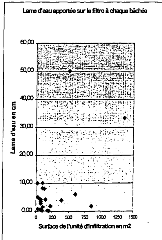
Graphique 10 : Hauteur de la lame d'eau par bâchée en fonction de la surface du filtre
