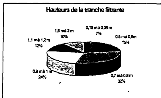
Graphique 9 : Hauteur de la tranche filtrante
