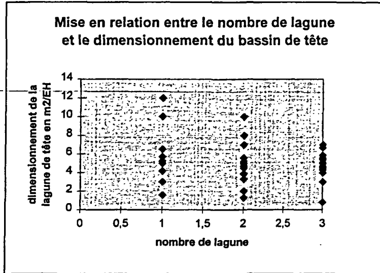
Graphique 4 : Relation entre la dimension de la lagune de tête et le nombre de bassins composant l'étage lagunage
