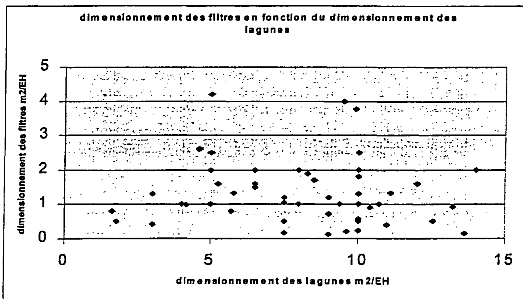
Graphique 6 : Dimensionnement des filtres comparé au dimensionnement des lagunes
