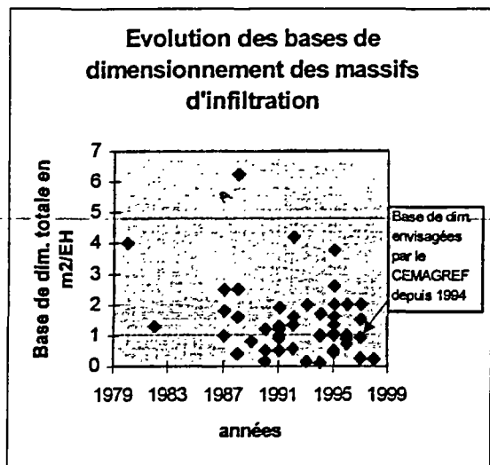
Graphique 5 : Evolution des bases de dimensionnement des massifs d'infiltration
