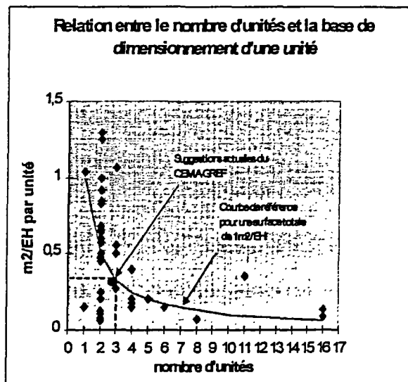
Graphique 8 : Relation entre le nombre d'unités d'infiltration et le base de dimensionnement d'une unité
