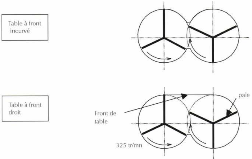
Figure 5.15 – Schéma des deux types de tables d'épandage utilisés
