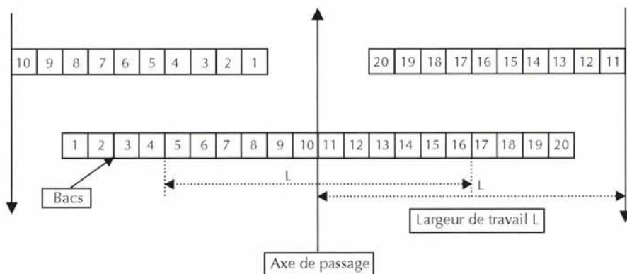
Figure 2.3 – Simulation de passages tous les 6 m pour un épandage va-et-vient
