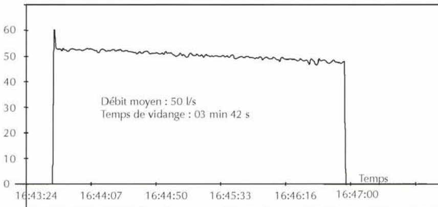
Figure 3.2 – Répartition longitudinale d'une tonne à lisier
