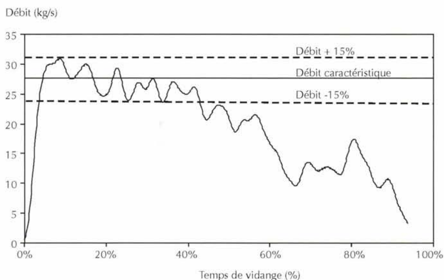
Figure 5.1 – Courbe de variation du débit durant le temps de déchargement (épandeur Rock Silex 2 )
