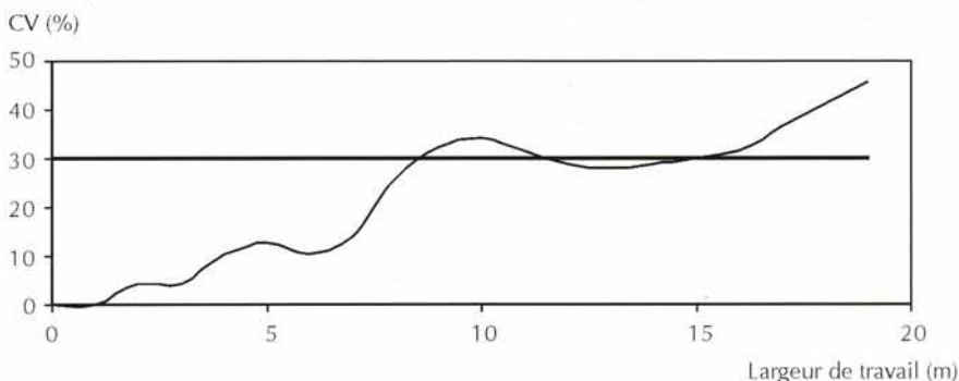
Figure 5.7 – Influence de la largeur de travail sur la valeur des coefficients de variation
