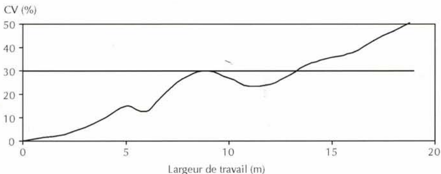
Figure 5.2 – Influence de la largeur de travail sur la valeur des coefficients de variation (épandeur Rock Silex 2).
