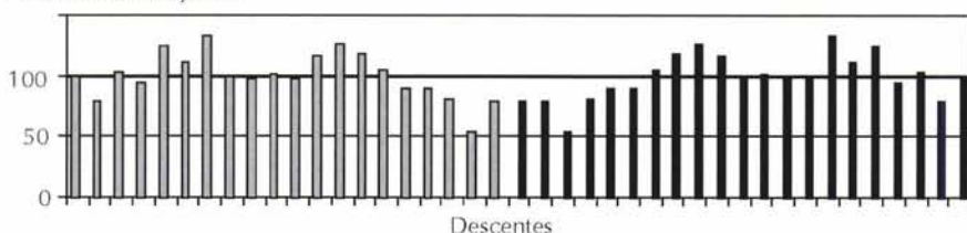
Figure 3.7 – Répartition de la rampe à pendillards (la mesure a été effectuée sur une demi-rampe uniquement).
