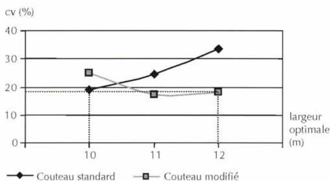
Figure 5.5 – Influence du type de couteaux sur la largeur optimale d'épandage (d'après M.N. Hansen)
