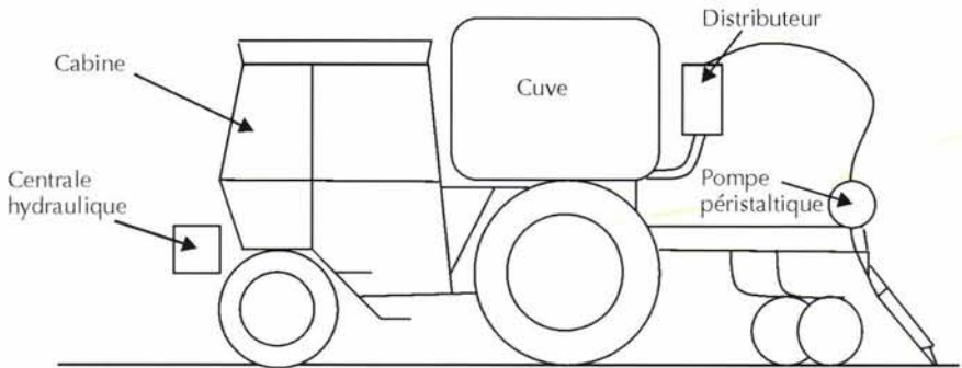
Figure 6.2 – Schéma général de l'épandeur danois pour parcelles expérimentales
