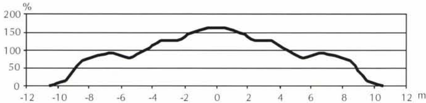
Figure 5.14 – Courbe de répartition déduite de l'observation de la nappe (cas d'une faible accumulation dans l'axe de passage)
