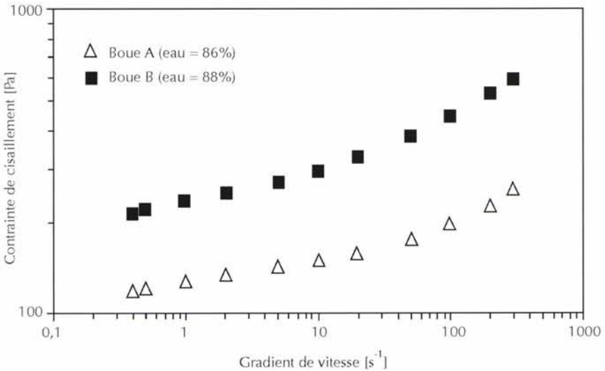
Figure 1.3 – Dans cet exemple, la boue la plus sèche est la plus fluide
