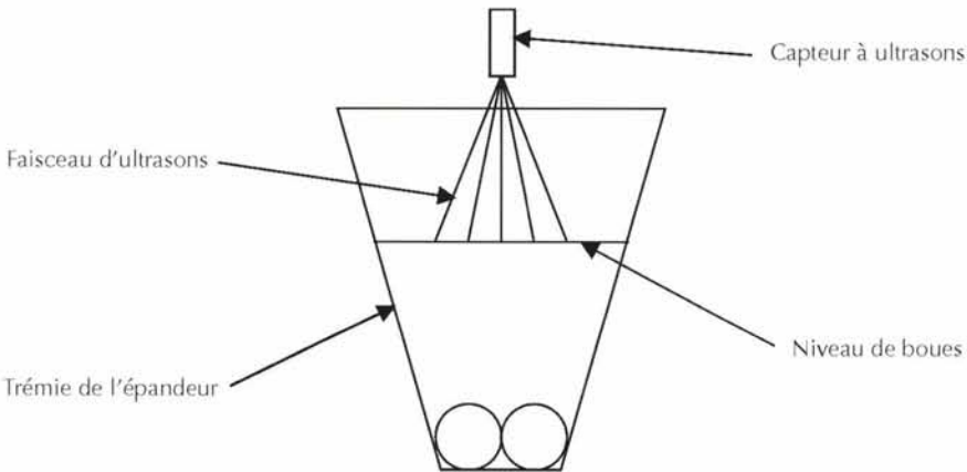
Figure 4.4 – Schéma de principe de mesure de débit par capteur.
