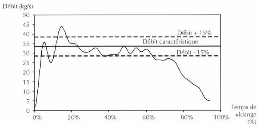
Figure 5.6 – Courbe de variation du débit durant le temps de déchargement
