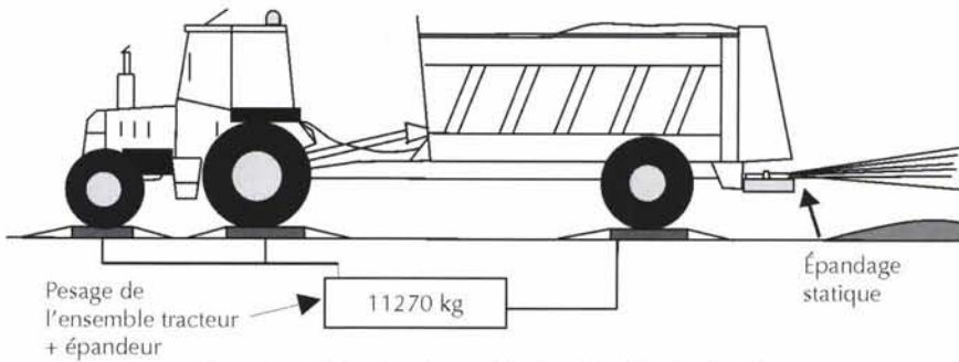
Figure 2.1 – Principe du test de répartition longitudinale
