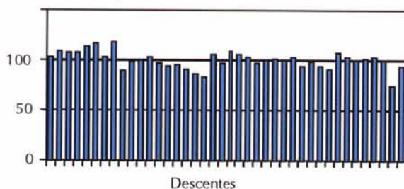
Figure 3.8 – Répartition satisfaisante d'une rampe à pendillards avec alimentation 150 mm.
