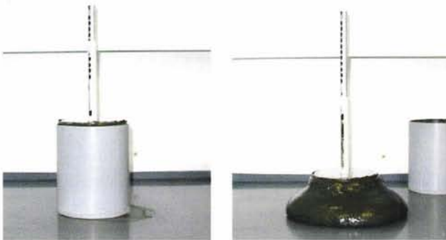
Photo 1.10 – Principe du test d'écrasement [J.-C. Baudez, Cemagref]
