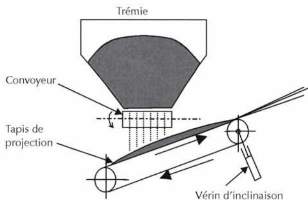
Figure 6.1 – Principe de fonctionnement de la machine d'épandage de compost par projection latérale
