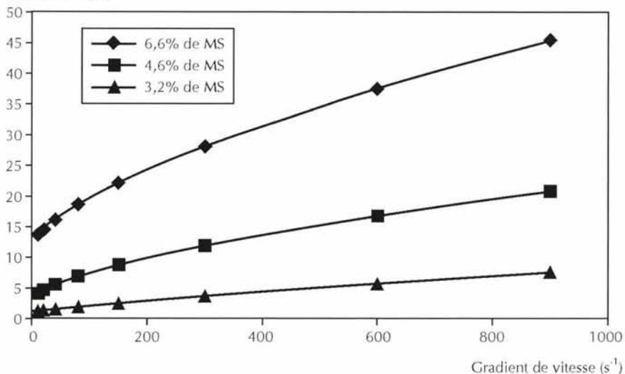
Figure 1.2 – Variation des caractéristiques d'écoulement suivant le taux de matière sèche
