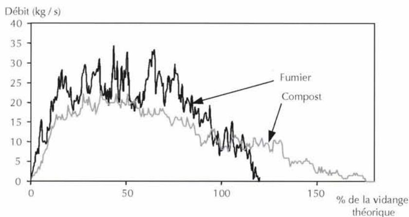
Figure 5.4 – Courbes de répartition longitudinale pour un fumier brut et un compost
