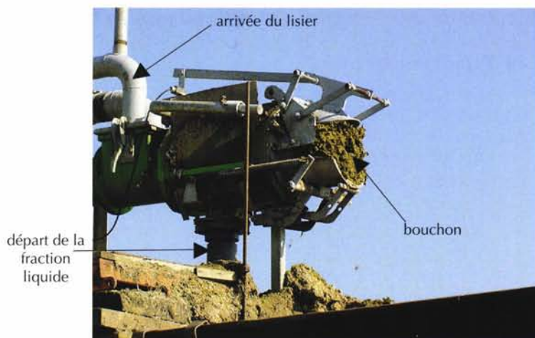
Photo 3.5 – Séparateur à vis en fonctionnement [F. Thirion, Cemagref]
