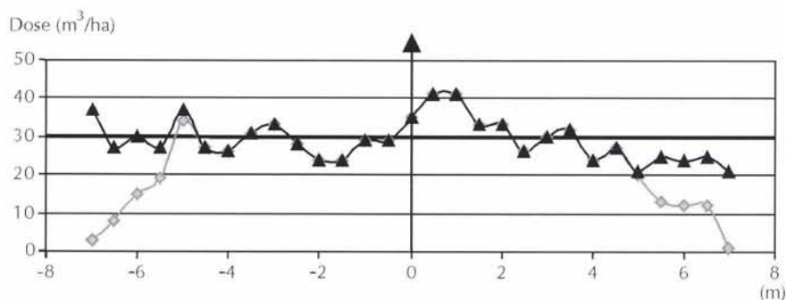
Figure 3.4 – Mesure de répartition avec une rampe à buses de 12 m, d'après F. Delaporte
