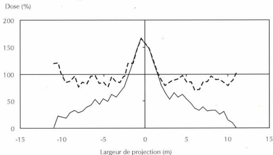
Figure 5.3 – Courbe de répartition transversale et simulation de passages tous les 12 m (épandeur Rock Silex 2)
