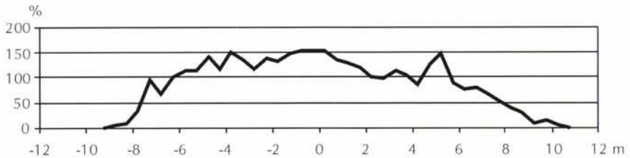
Figure 5.12 – Courbe de répartition réelle de l'épandeur présenté sur la photo 5.5
