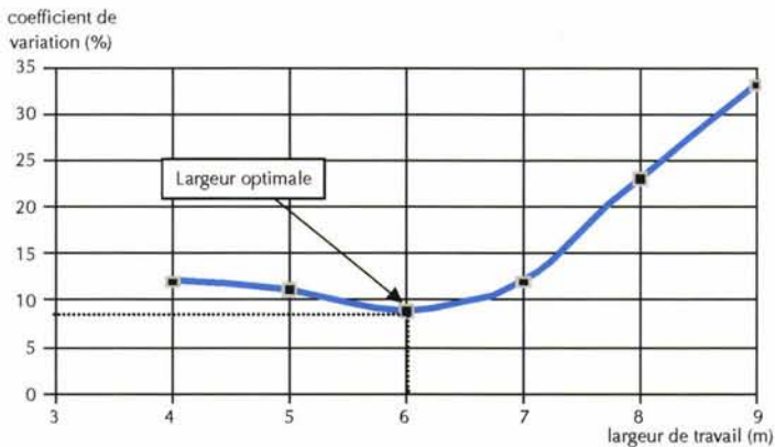
Figure 2.5 – Exemple d'évolution du coefficient de variation suivant la largeur de travail
