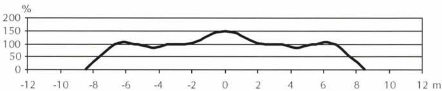
Figure 5.11 – Courbe de répartition déduite de la nappe théorique
