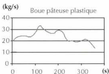
Figure 4.2 – Influence de la consistance de la boue sur la régularité longitudinale
