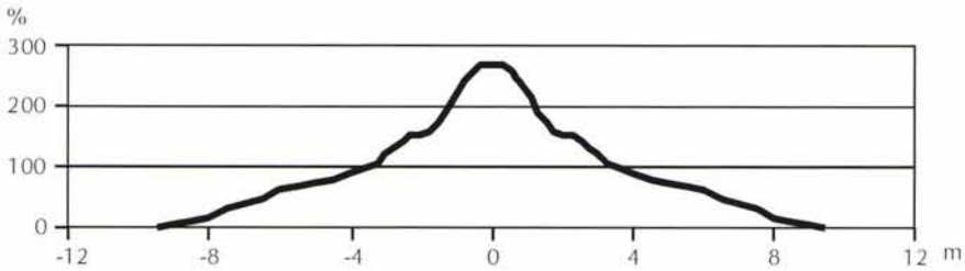
Figure 5.17 – Courbe de répartition déduite de l’observation de la nappe (cas d’une table à front droit)
