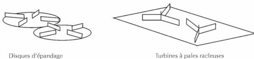
Figure 5.21 : Schéma des deux types de rotors pour table d'épandage.
