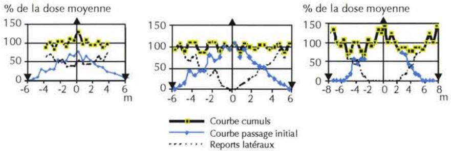
Figure 2.4 – Courbes de répartition pour des largeurs de travail de 4, 6 et 8 m
