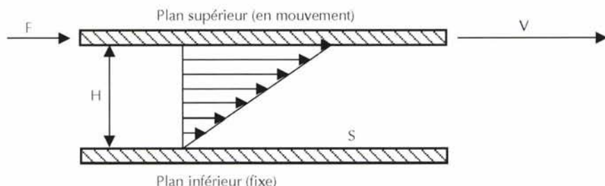
Figure 1.1– Profil de vitesses lors d'un cisaillement simple imposé à un fluide confiné entre deux plans solides
