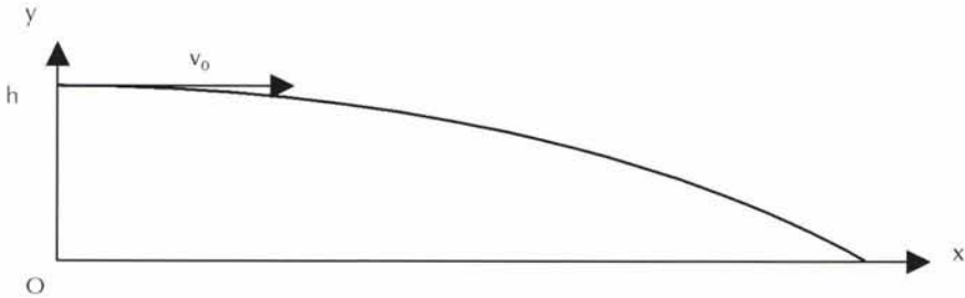
Figure 5.10 – Trajectoire du produit éjecté par la table d'épandage
