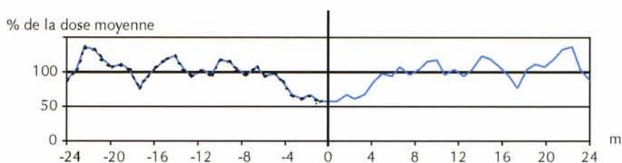
Fig. 3.1 – Répartition de la rampe (La mesure a été effectuée sur une demi-rampe uniquement)
