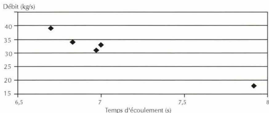
Figure 3. 3 – Débit de la tonne à lisier en fonction de la viscosité du liquide (d'après Malgreryd et Wetterberg)
