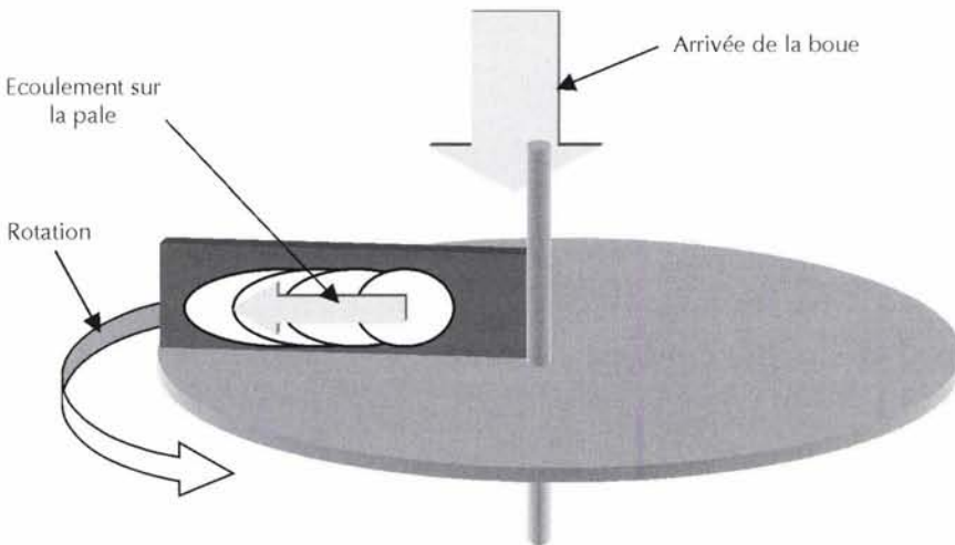
Figure 4.6 – Schéma de principe du fonctionnement du disque d'épandage.
