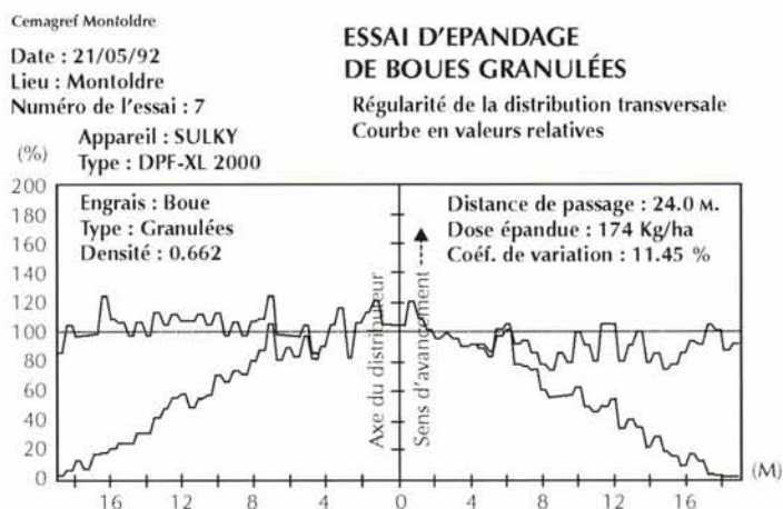
Figure 5.23 – Courbe de répartition transversale pour une largeur de travail de 24 m
