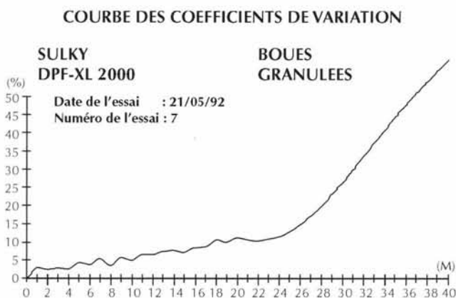
Figure 5.22 – Influence de la largeur de travail sur la valeur des coefficients de variation.
