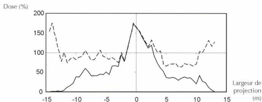
Figure 5.8 – Courbe de répartition transversale et simulation de passages tous les 14 m (épandeur Tebbe HKS 100)
