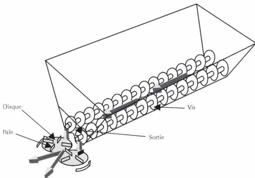
Figure 4.1 – Principe de fonctionnement des épandeurs à boues pâteuses
