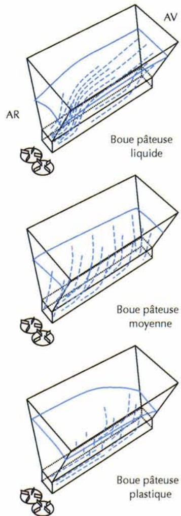
Figure 4.3 – Schéma des écoulements simulés de trois boues différentes
