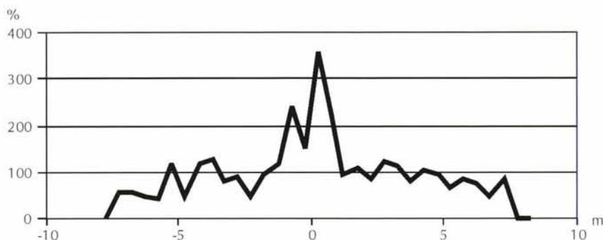
Figure 5.20 – Courbe de répartition mesurée avec une table à 4 rotors
