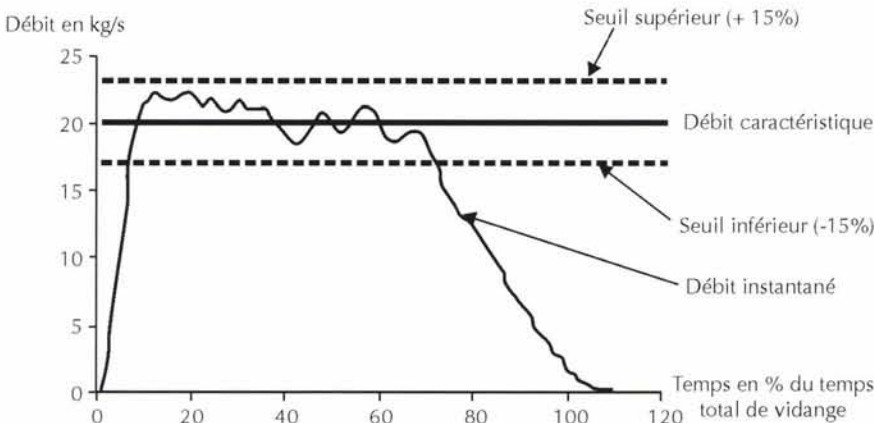
Figure 2.2 – Courbe de variation du débit durant le temps de déchargement
