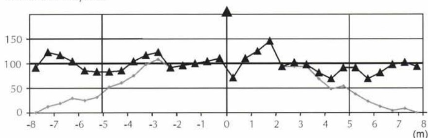
Figure 4.5 – Courbe de répartition transversale d'un épandeur de boues pâteuses
