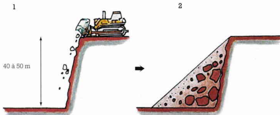
Figure 65 : Talutage depuis le haut par déversement [75].
