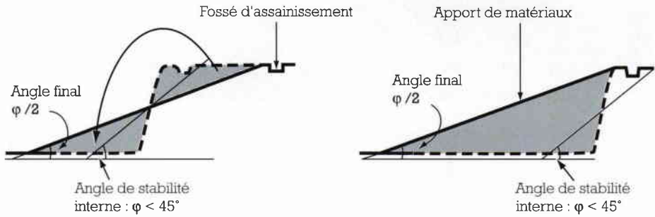
Talutage par équilibre déblais-remblais
