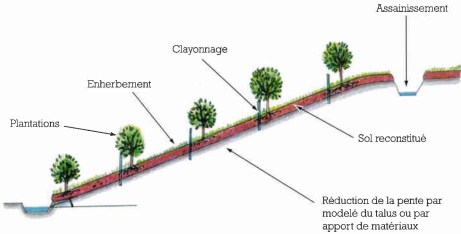
Figure 74 : Fossé d'assainissement en tête de talus [TPG 2].
