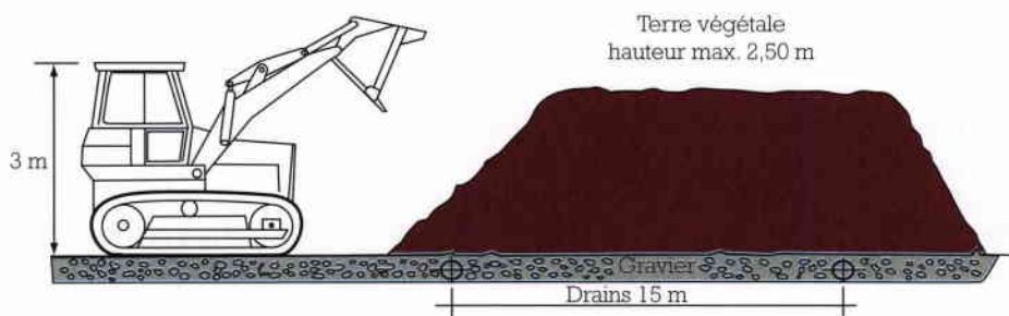
Figure 16 : Préparation d'un site de stockage sur un sol imperméable (d'après [62a]).
