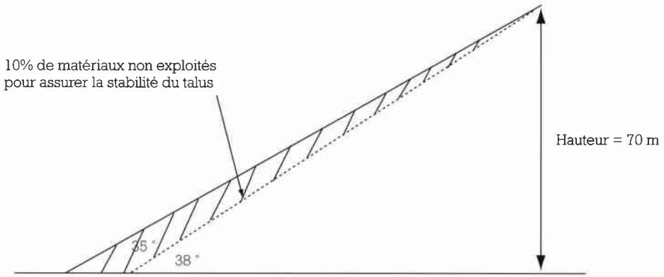
Figure 62 : Réduction de la pente d'un talus et perte en matériau [F14 Mo].
