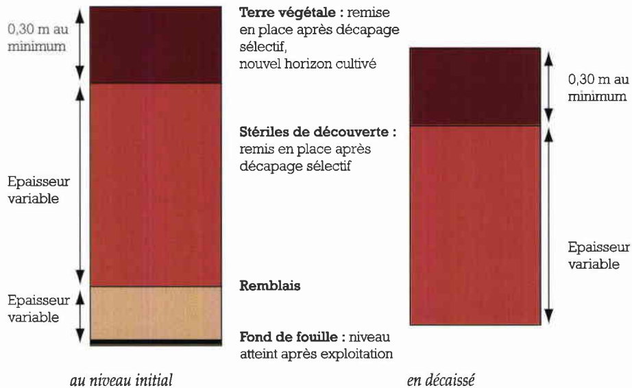
Figure 32 : Schéma d'un profil de sol reconstitué.
