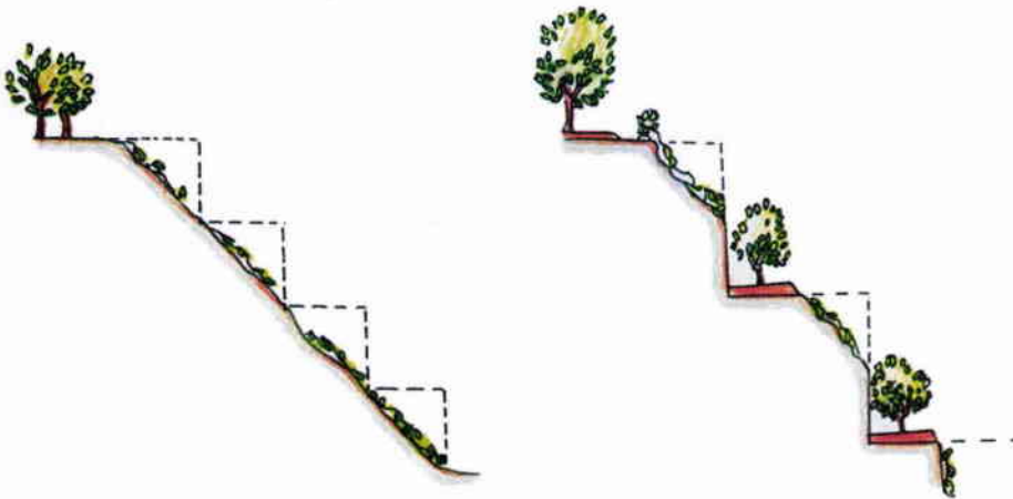
Figure 64 : Profils rectifiés par écrêtage de gradins [75].
