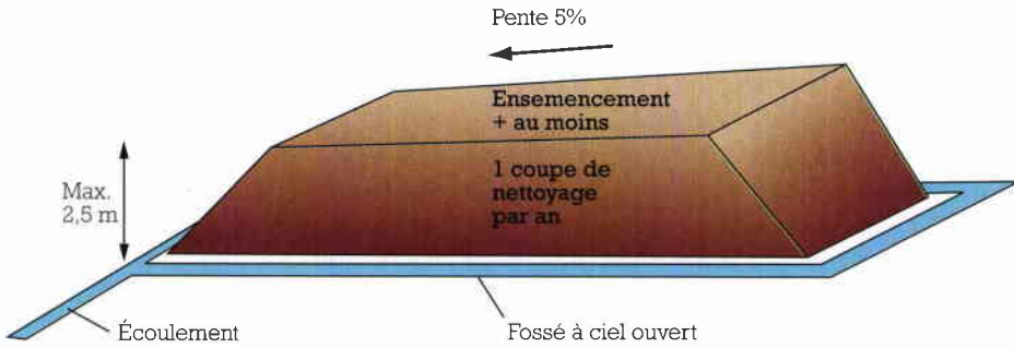
Figure 17 : Schéma d'un stock de terre végétale (d'après [62a]).
