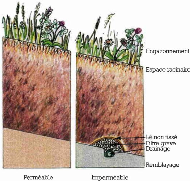
Figure 36 : Réalisation d'un collecteur sur un remblai imperméable [5].
