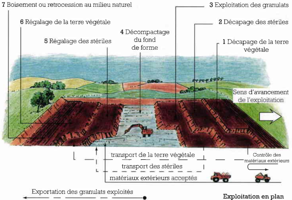
Figure 29 : Schéma d'un réaménagement forestier à l'avancée.
