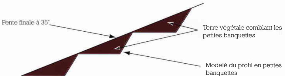
Figure 71 : Modelé du profil du talus et comblement par de la terre végétale.
