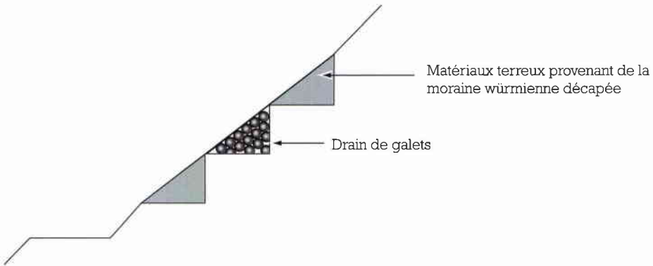
Figure 75 : Réalisation des drains en galets à flanc de pente [F14 Mo].
