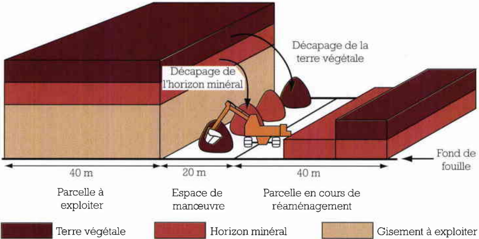
Figure 30 : Schéma de décapage pour faciliter les manœuvres.
