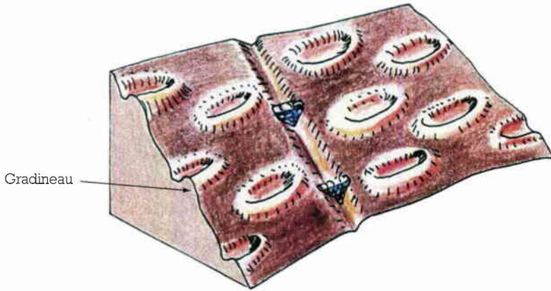
Figure 85 : Réalisation de petits gradins sur une pente [27].
