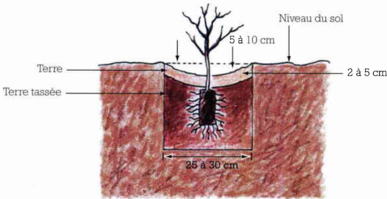
Figure 55 : Façonnage en cuvette d'une plantation [27].
