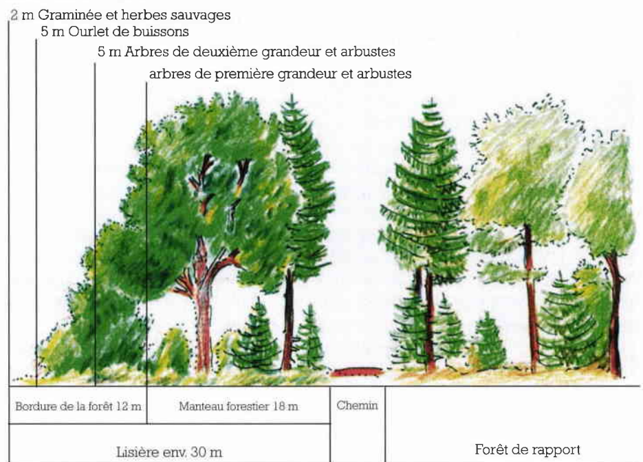
Figure 50 : Constitution d'une lisière en bordure de peuplement de rapport 125 (d'après [5]).
