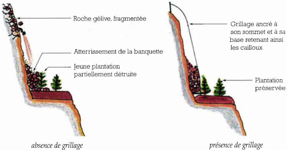
Figure 68 : Protection contre les chutes de pierre du front de taille [75].
