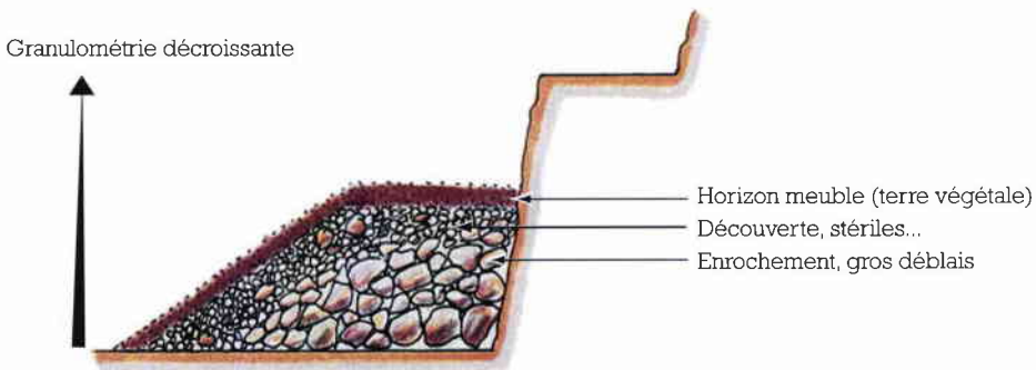
Figure 76 : Composition granulométrique optimale d'un talus en pied de front de taille [75].
