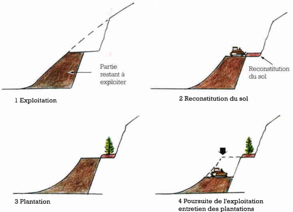
Figure 61 : Végétalisation d'une banquette en cours d'exploitation [75].
