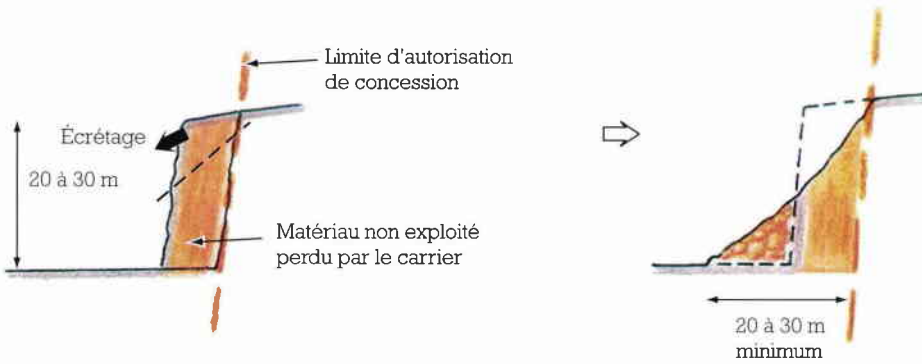
Figure 63 : Ecrêtage d'un front de taille engendrant une perte de matériau exploitable [75].
