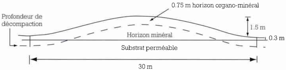
Figure 40 : Modelé du terrain en billons (d'après [92]).
