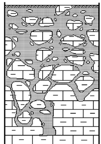
Figure 13. Altérites mixtes
