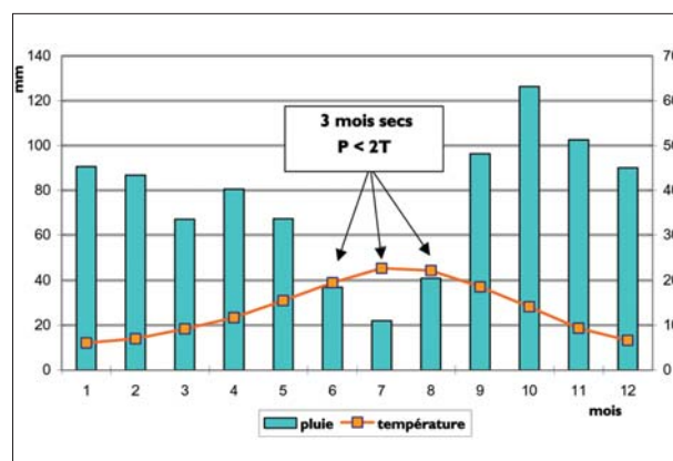
Figure 6. Courbe ombrothermique de Brignoles : moyenne 1961-1996
