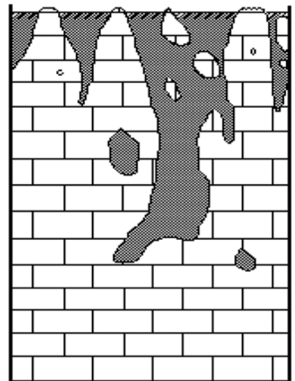
Figure 12. Altérite de dissolution biochimique de la roche
