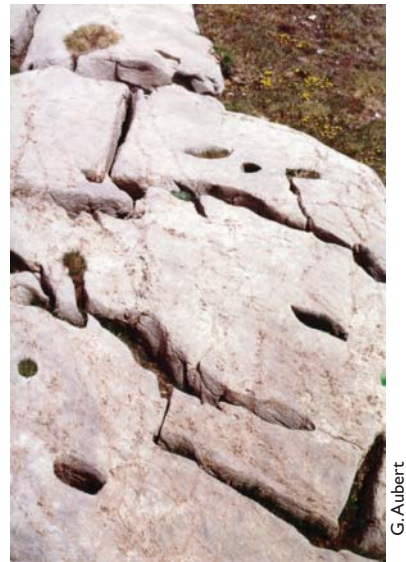
Formes caractéristiques d'un lapiaz
