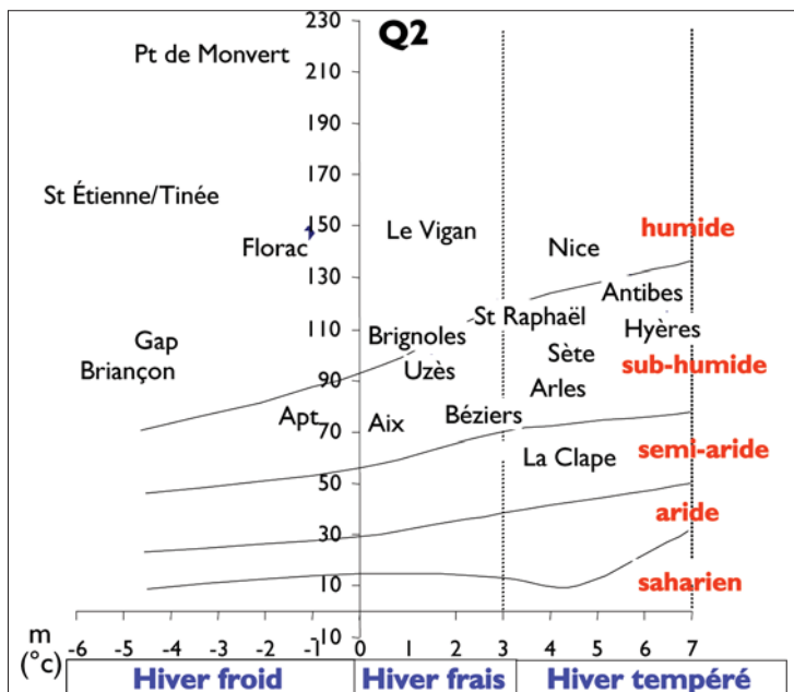
Figure 7. Climagramme d'Emberger
