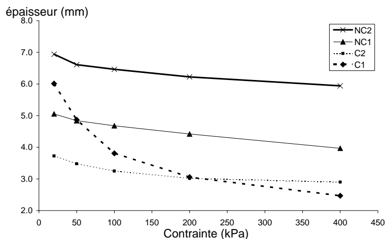
Figure 2. Epaisseurs des produits après 2 minutes de fluage
