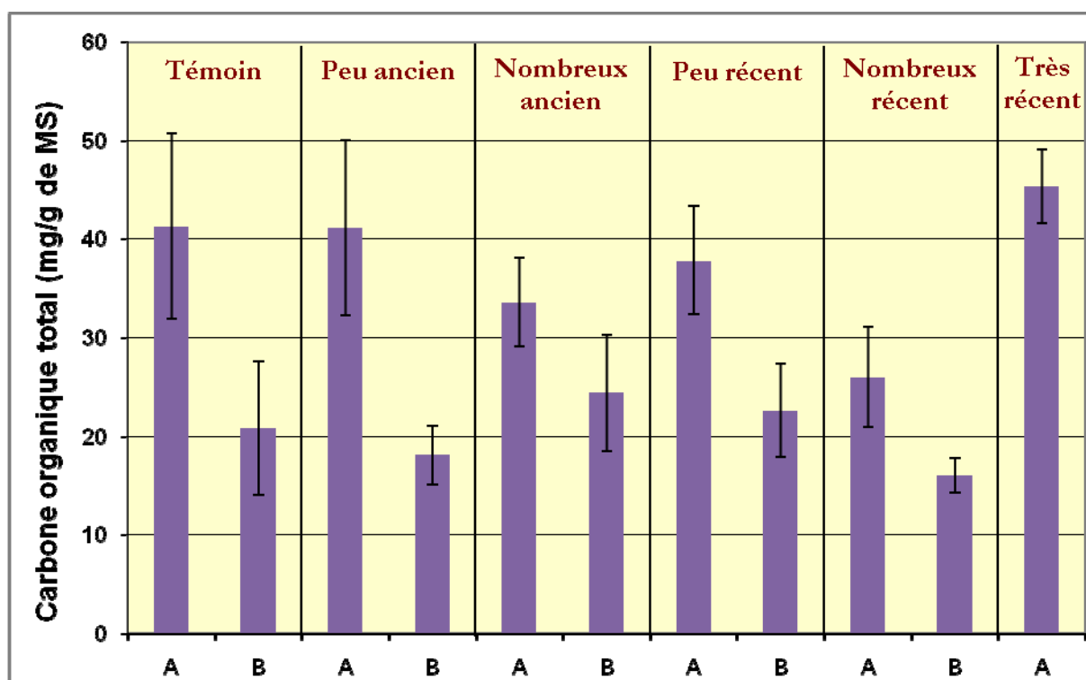
Figure 2 : Teneur en Carbone Organique Total dans les sols (A : 0 à -5 cm; B : -5 à -15 cm). Résultats moyens obtenus sur 5 échantillons de sols par type de feux ; intervalles de confiance, P=0,05.
