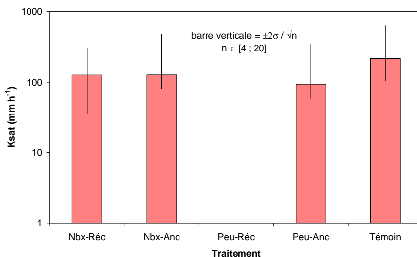
Figure 3 : valeurs de K_{sat} ( mm\ h^{-1} ) en fonction des traitements.
