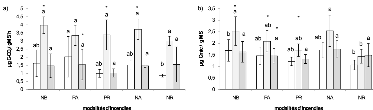
Figure 5 : Respiration basale (a) et biomasse microbienne (b) de sols prélevés sur les parcelles incendiées et incubées avec, soit des apports de feuilles sénescées broyées de ciste de Montpellier (-FB, barres grisées claires), soit des tanins condensés extraits de ce ciste, et purifiés (-Tc, barres grisées foncées), soit avec aucun apport (-C, barres blanches). Les modalités d'incendies en abscisse sont NB (non brûlées), PA (peu anciens), NA (nombreux anciens), PR (peu récents) et NR (nombreux récents). Valeurs moyennes \pm écart type (N = 5). Pour une série d'échantillons -C, -FB, ou -Tc, et par variable, les moyennes surmontées d'une même lettre minuscule ne sont pas significativement différentes au seuil de p < 0,05 (test de Tukey). Le signe * indique un effet significatif (test t) de l'amendement en feuilles broyées ou en tanins condensés sur la modalité précisée en abscisse.
