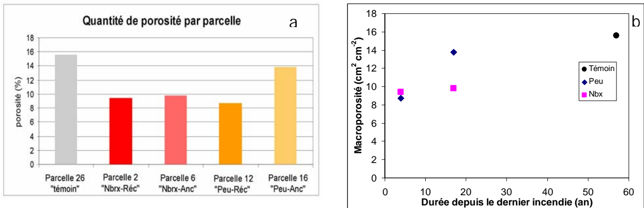
Figure 7 : évolution de la macroporosité en fonction de la modalité (a) et en fonction de la durée depuis le dernier incendie (b).
