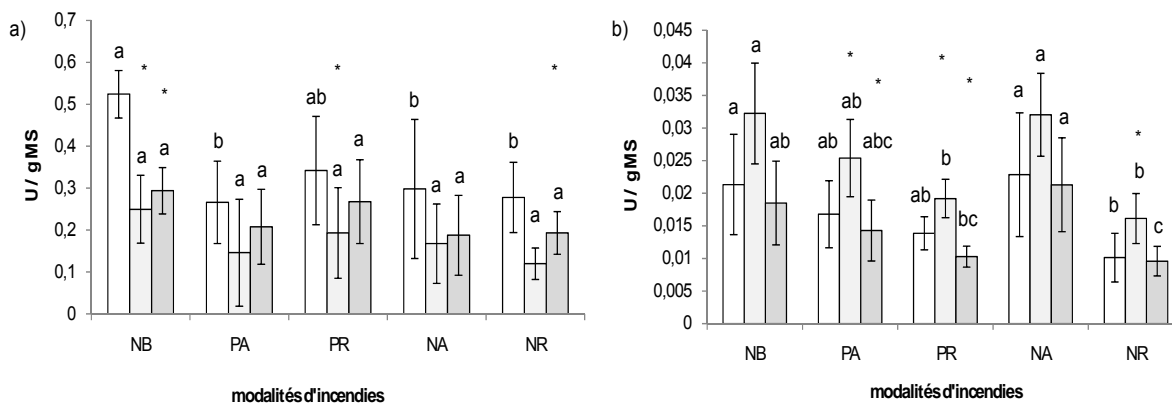
Figure 6 : Activités phénol-oxydase (a) et \beta -glucosidase (b) de sols prélevés sur les parcelles incendiées, et incubés avec soit des apports de feuilles sénescentes broyées de ciste de Montpellier (barres grisées claires), soit des tanins condensés extraits de ce ciste et purifiés (barres grisées foncées), soit avec aucun apport (barres blanches). Les modalités d'incendie en abscisse sont NB (non brûlées), PA (peu anciens), NA (nombreux anciens), PR (peu récents) et NR (nombreux récents). Valeurs moyennes \pm écart type (N = 5). Pour une série d'échantillons -C, -FB, ou -Tc, et par variable, les moyennes surmontées d'une même lettre minuscule ne sont pas significativement différentes au seuil de P<0,05 (test de Tukey). Le signe * indique un effet significatif (test t) de l'amendement en feuilles broyées ou en tanins condensés sur la modalité précisée en abscisse.
