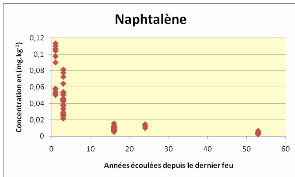
Figure 5: Evolution de la teneur en naphtalène après feux de forêt
