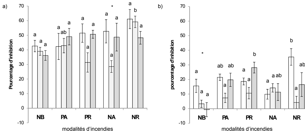
Figure 7 : Pourcentage d'inhibition des activités phénol-oxydase (a) et \beta -glucosidase (b) mesuré sur les sols des parcelles incendiées et incubés avec, soit des apports de feuilles sénescentes broyées de ciste de Montpellier (-FB, barres grisées claires), soit des tanins condensés extraits de ce ciste et purifiés (-Tc, barres grisées foncées), soit avec aucun apport (-C, barres blanches). Les modalités d'incendies en abscisse sont NB (non brûlées), PA (peu anciens), NA (nombreux anciens), PR (peu récents) et NR (nombreux récents). Valeurs moyennes \pm écart type (N = 5). Pour une série d'échantillons -C, -FB, ou -Tc, et par variable, les moyennes surmontées d'une même lettre minuscule ne sont pas significativement différentes au seuil de P < 0,05 (test de Tukey). Le signe * indique une différence significative (test t) entre le pourcentage d'inhibition des sols -FB et -C ou -Tr et -C sur la modalité précisée en abscisse.
