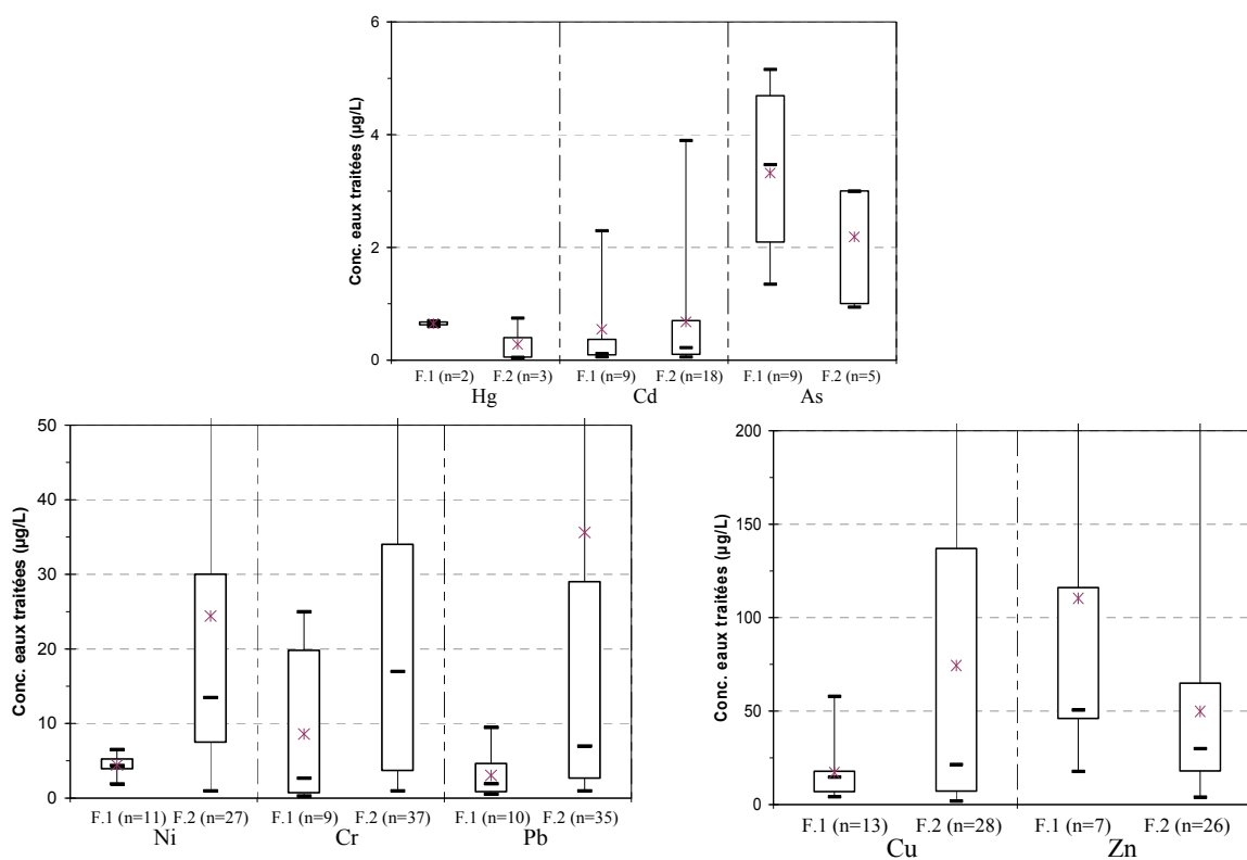
Figure 4 : Concentrations en métaux dans les eaux résiduaires traitées (µg/L) de la base de données et comparaison des données de fiabilité 1 et 2 (F.1 ; F.2) ; n : nombre de données > LQ
