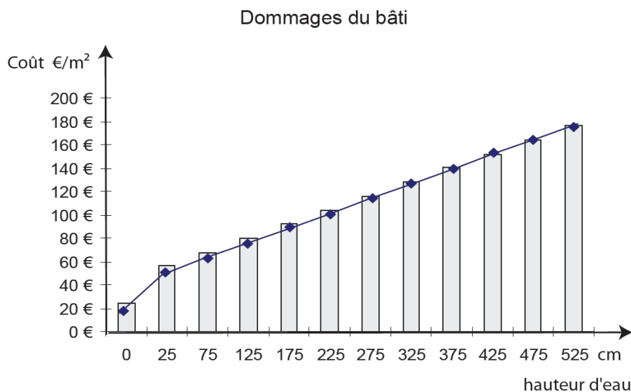
FIG. 5.3 – Courbe de dommages au bâti en fonction de la submersion
