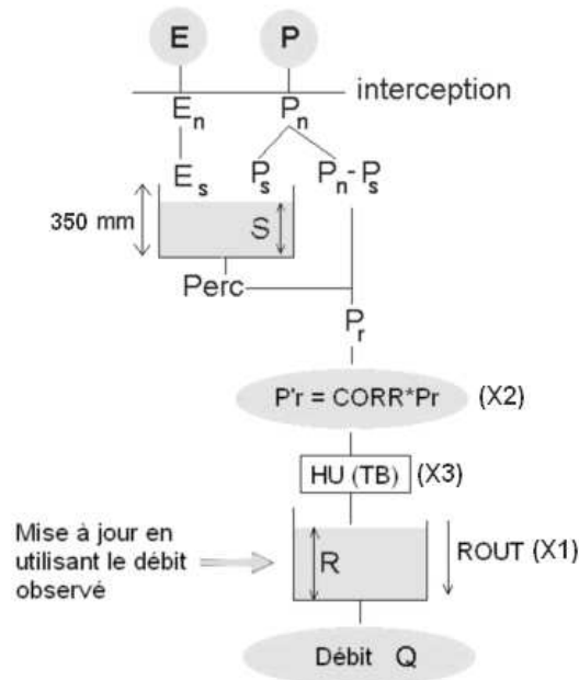
Figure 8 : Structure du modèle GR3P utilisé dans l'étude et ses trois paramètres libres : X1 (ROUT), X2 (CORR) et X3 (TB) (d'après Tangara, 2005)
