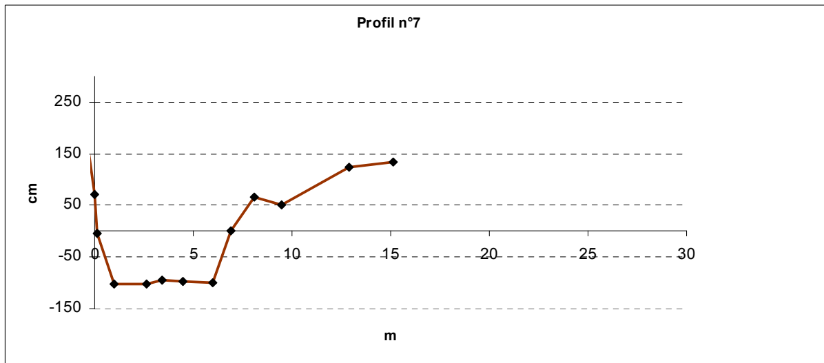
Figure 9 : Profil en travers 7.
