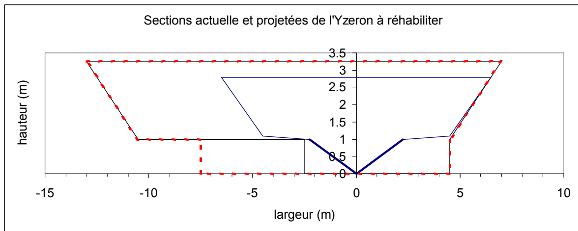
Figure 1 : détail des sections testées pour l'étude du débit seuil de charriage.
