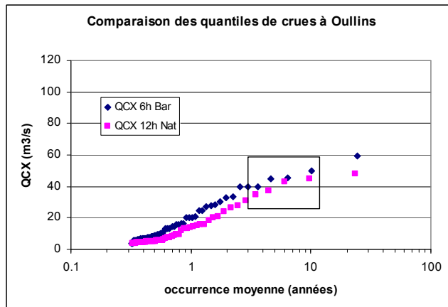
Figure 3 : Illustration de l'augmentation de la durée des crues à Oullins par effet de laminage.
