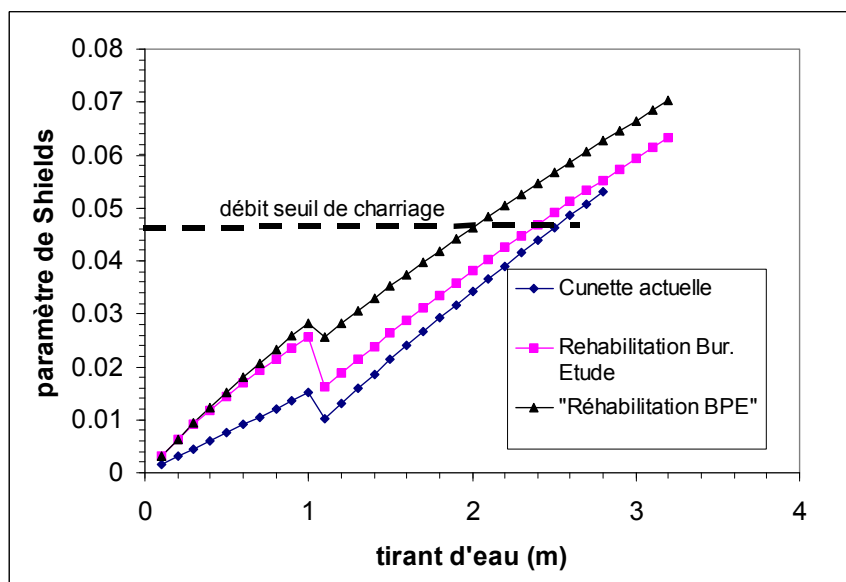
Figure 3 : Détection du tirant d'eau de charriage dans l'Yzeron à Oullins pour la situation actuelle et deux hypothèses d'élargissement.
