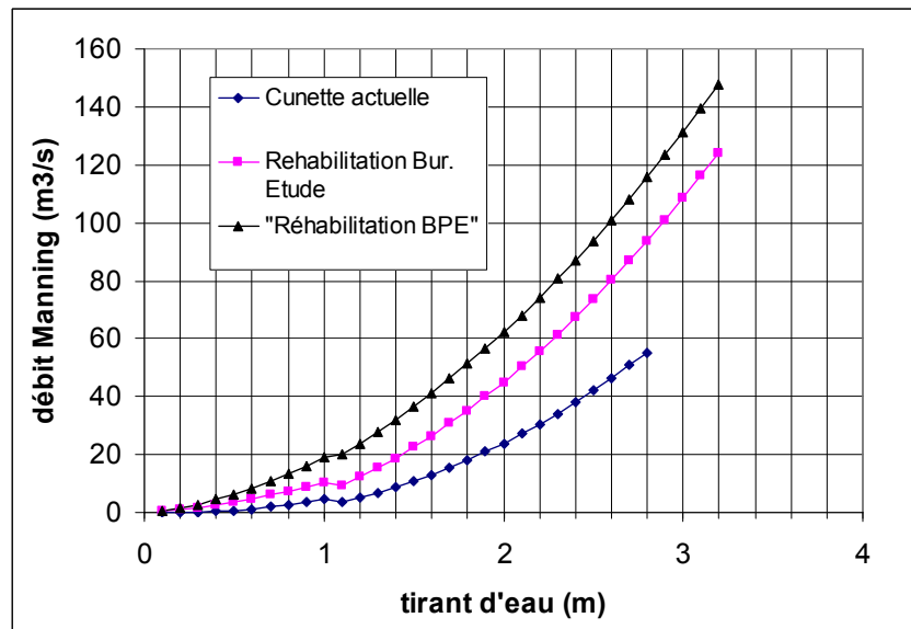
Figure 2 : Evolution des débits en fonction du tirant d'eau dans l'Yzeron au niveau d'Oullins (situation actuelle et deux hypothèses d'élargissement)
