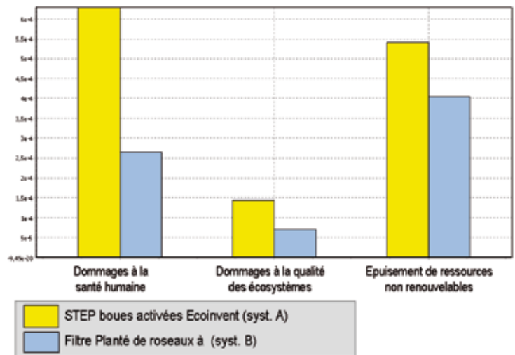
Exemple de résultats d'ACV exprimés avec des indicateurs de dommages correspondant aux trois aires de protection de l'ACV
