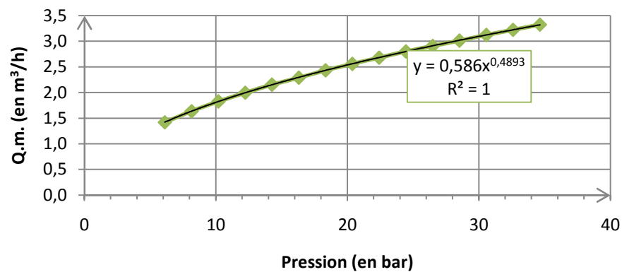
Loi débit-pression (JDW In-line Hydrogol)
