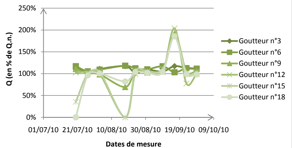
Evolution du débit au cours du temps (JDW In-line Hydrogol)
