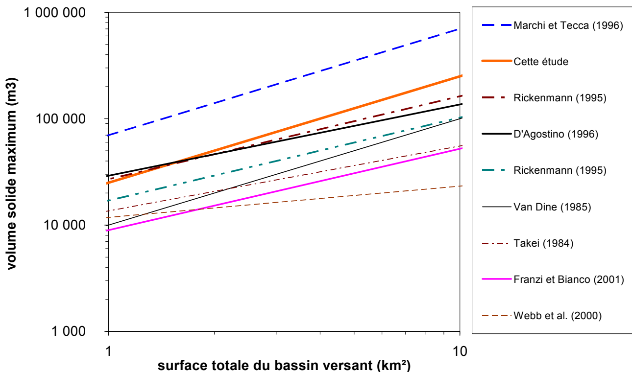
Figure 16. Comparaison de la relation V_{\max} = 25000.S proposée dans cette étude avec des relations similaires publiées par d'autres auteurs
