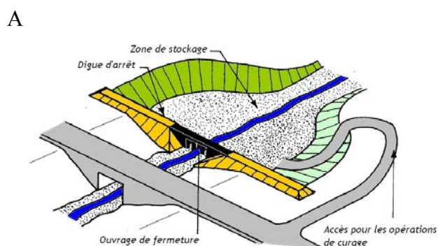
Figure 2. (A) Schéma de principe d'une plage de dépôt (Van Dine, 1996) ; (B) opération de curage mécanique d'une plage de dépôt sur un torrent isérois (photo : Pascal Diot)
