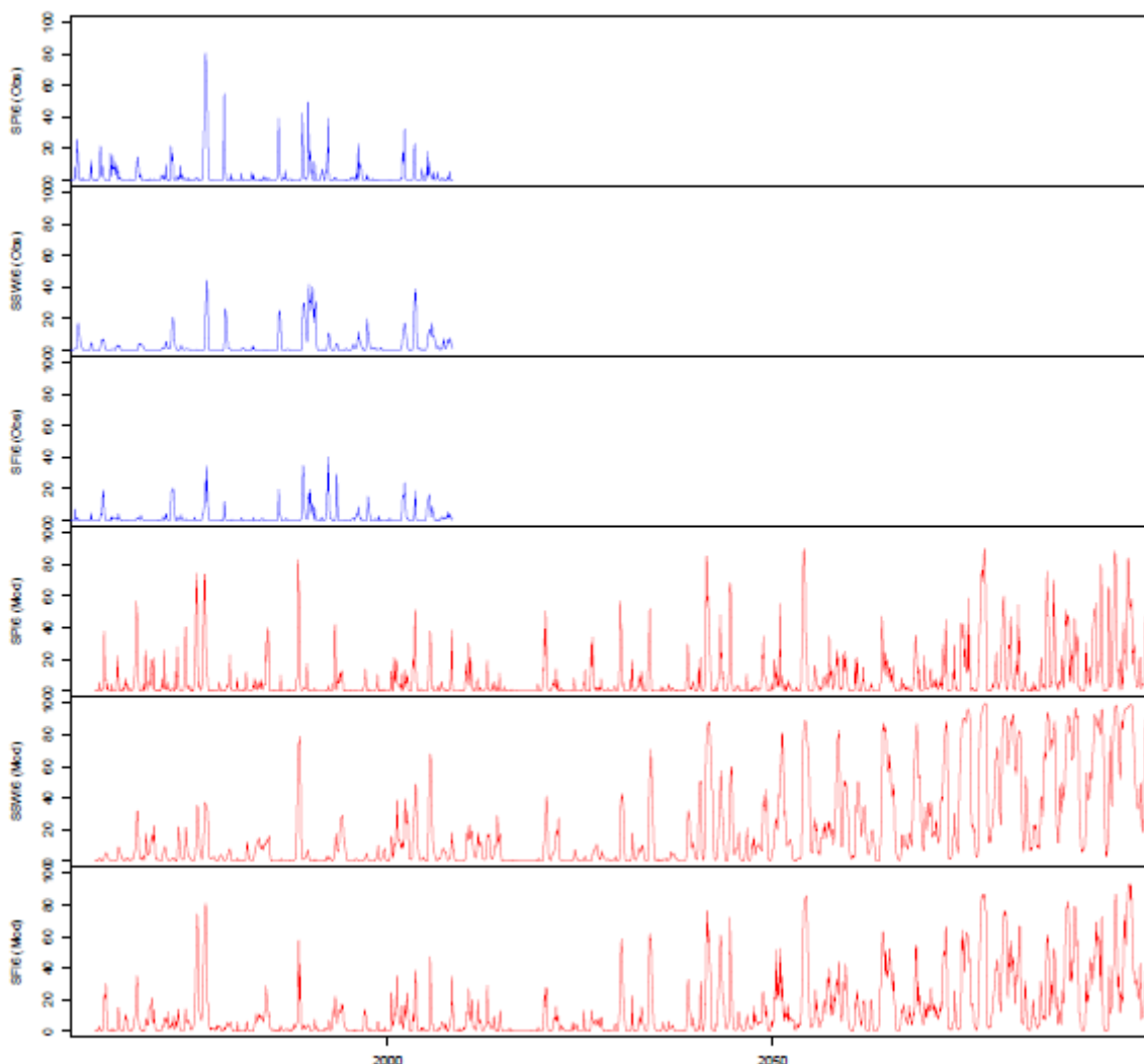
Figure 2-1 Proportion de la surface de la France affectée par une sécheresse sévère (échelle de temps 6 mois et seuil 5%). En bleu, réanalyse SIM 1958-2008 (Obs). En rouge, simulation sur la période 1961-2099 (Mod). De haut en bas, sécheresses météorologiques (SPI), agricoles (SSWI) et hydrologiques (SFI).
