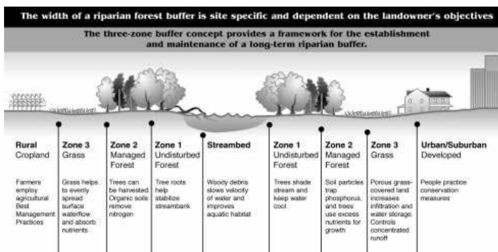
Figure 19 : Principe du dispositif à triple bande
