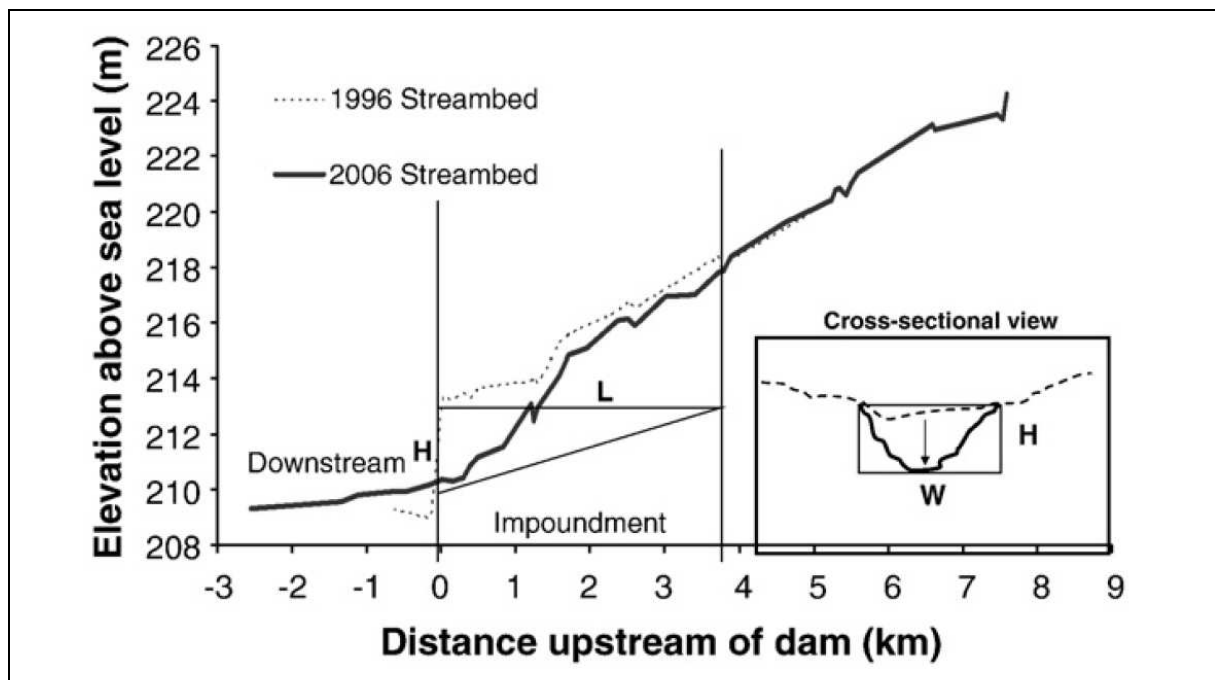
Figure 9 : exemple d'emprise d'une érosion régressive suite à l'effacement d'un seuil sur la Pine River (Burrough et al., 2009).
