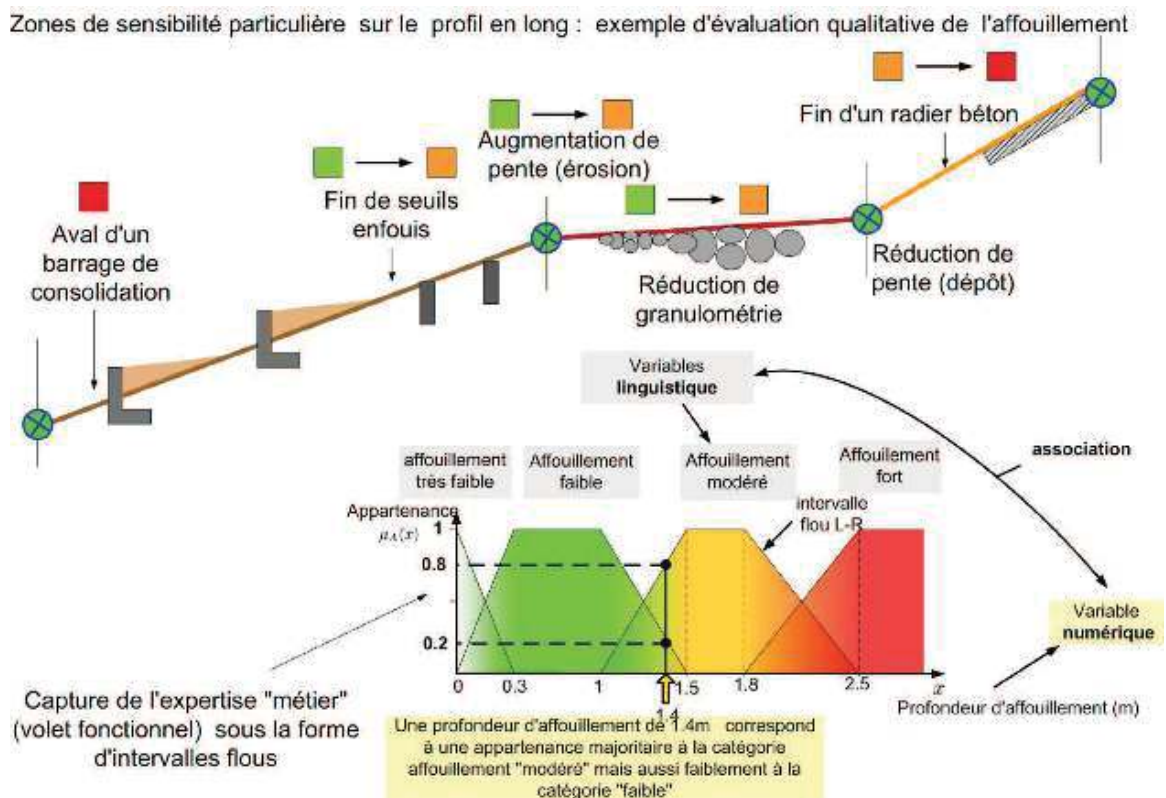
Figure 7. Evaluation qualitative de la sensibilité du lit à l'affouillement
