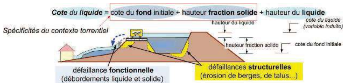
Figure 2. Défaillances structurales et fonctionnelles d'une digue de correction torrentielle
