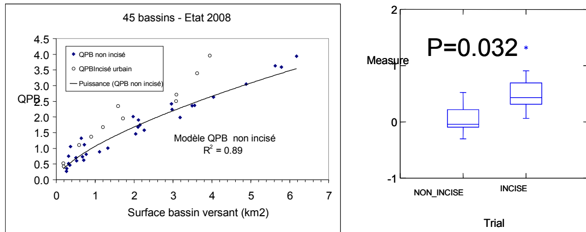
Figure 6.55: (gauche) Distribution des QPB périurbains pour les bassins à cours d'eau incisé (rond blanc) et non incisé (losange noir). La courbe représente le modèle de référence ajusté par les moindres carrés des stations non incisées. (droite) La déviation du QPB est calculée par différence au modèle.
