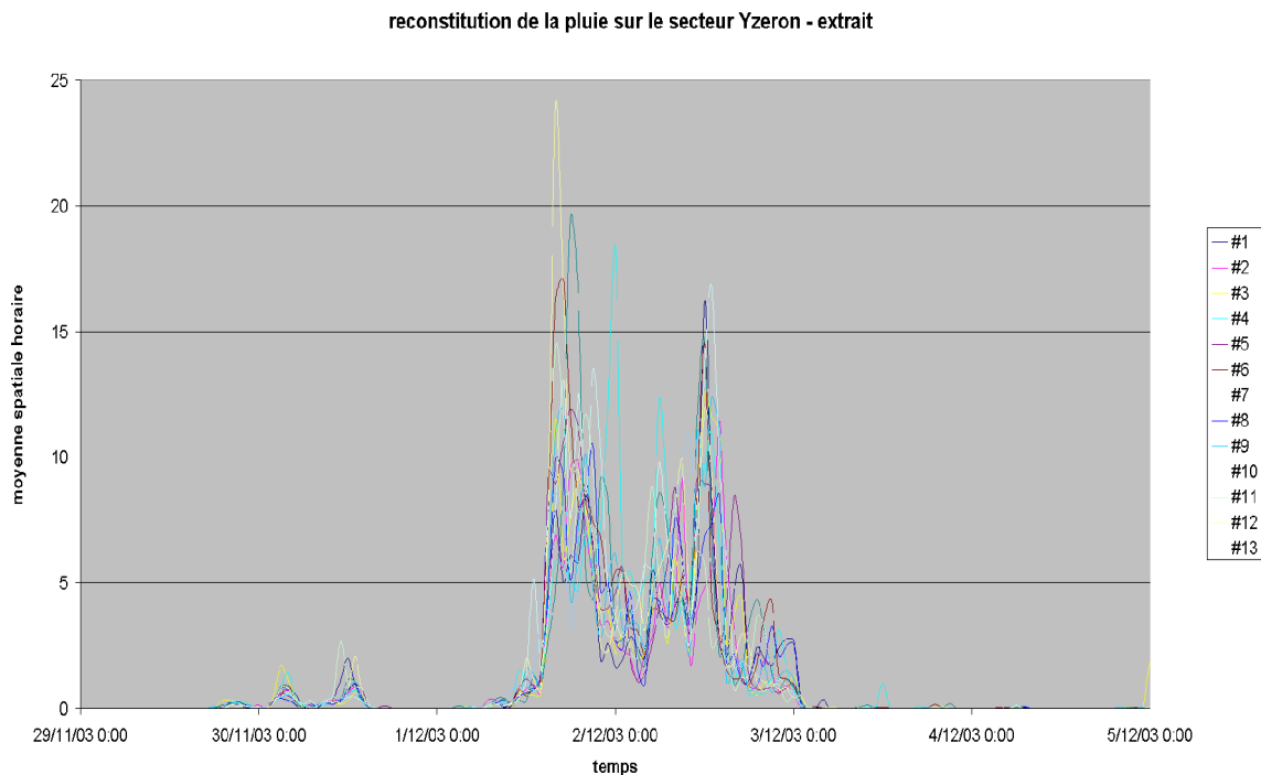
Figure 6.37: Reconstitutions de la pluie horaire relative à l'événement de décembre 2003. Ici, moyenne horaire de bassin, 13 membres. CV du cumul de l'événement 0.2
