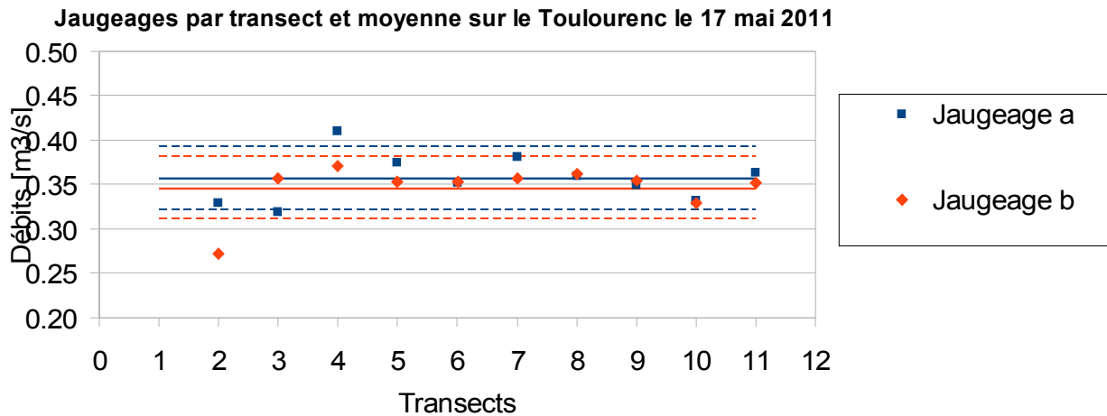
Fig. 14 : Jaugeages sur le Toulourenc, dépouillements à 3 points (Norme ISO 748)
