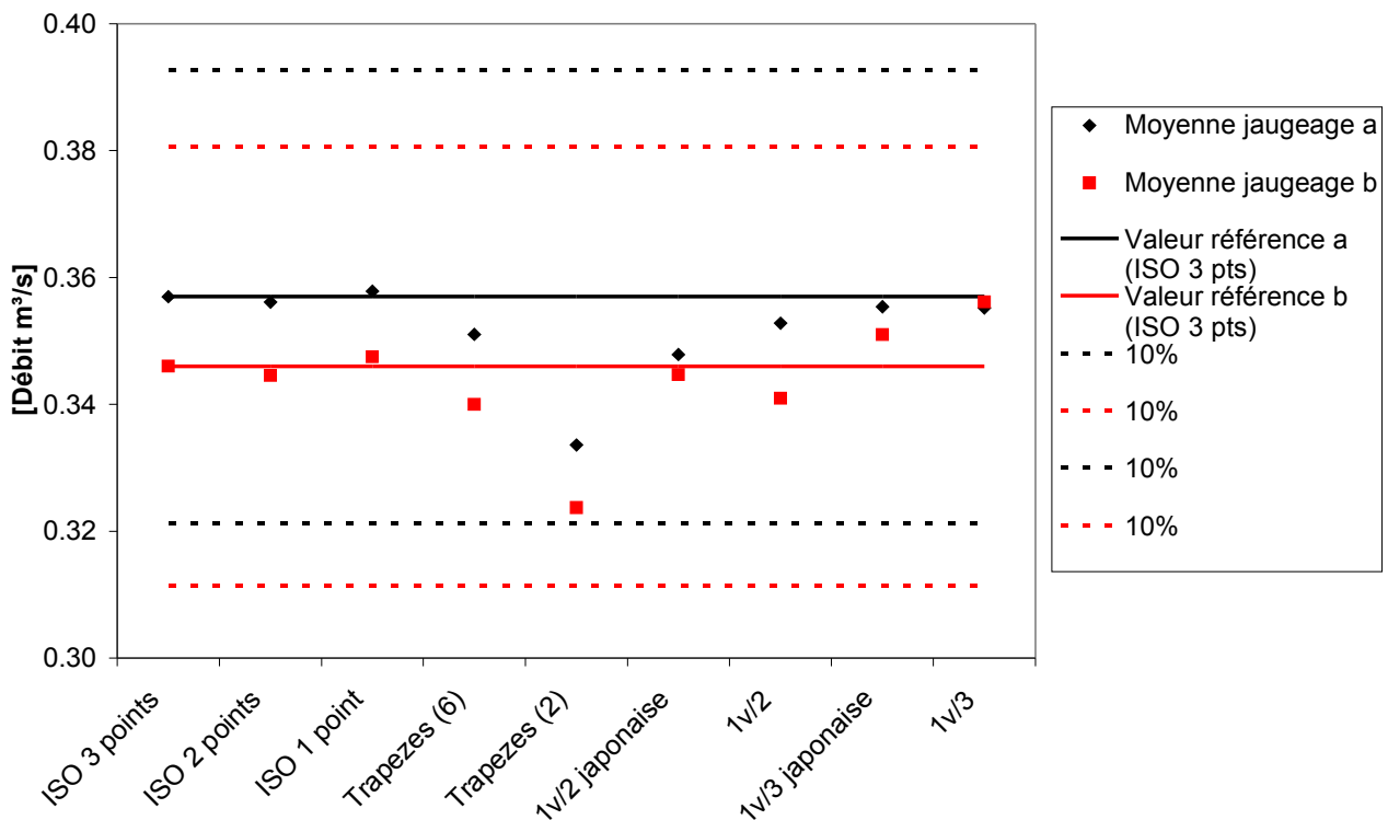
Fig. 15 : Moyenne des débits en fonction de la méthode de dépouillement sur le Toulourenc
