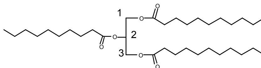
Figure 6. Exemple d'un triglycéride : le 1,2,3-tridecanoyl- sn -glycérol.
