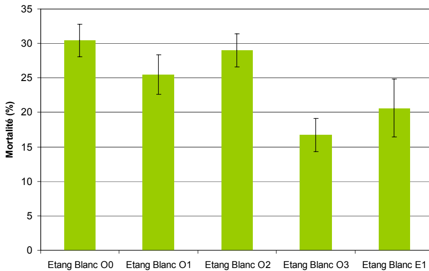
Figure 9 : % de diatomées mortes dans les échantillons
