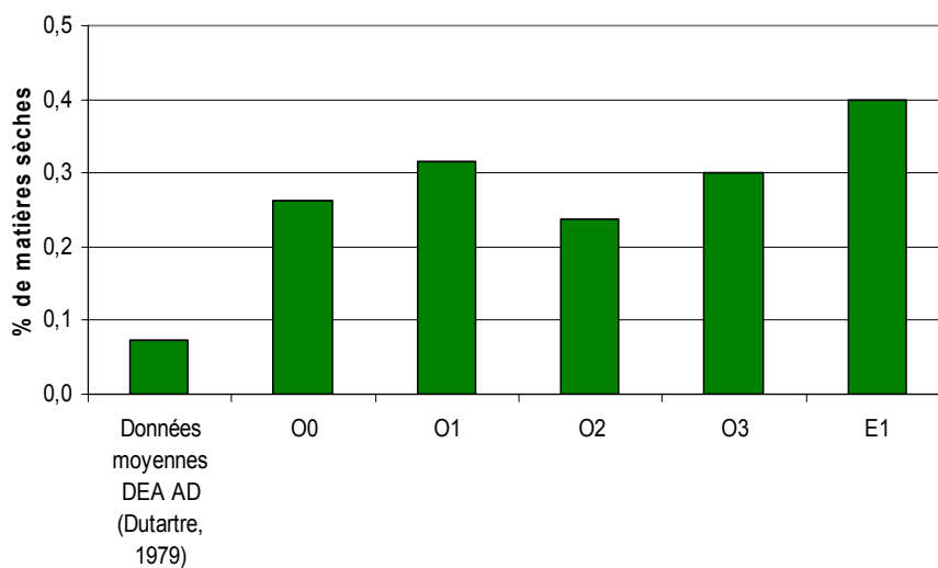
Figure 5 : Teneurs en phosphore des segments index des plantes dans les différentes stations (% des matières sèches)
