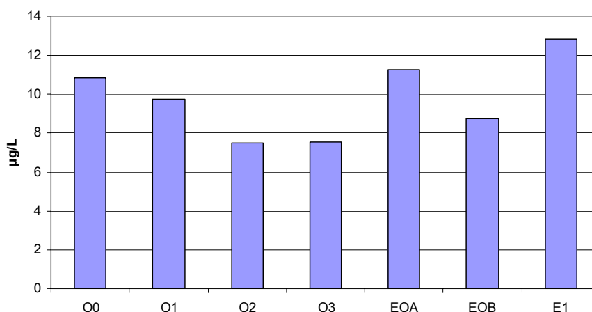
Figure 8 : Teneurs en pigments chlorophylliens des eaux de surface
