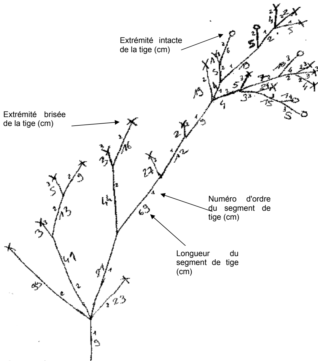
Figure 3 : Mesures sur l'architecture des pieds de lagarosiphon (exemple pied N° 2, station E1)
