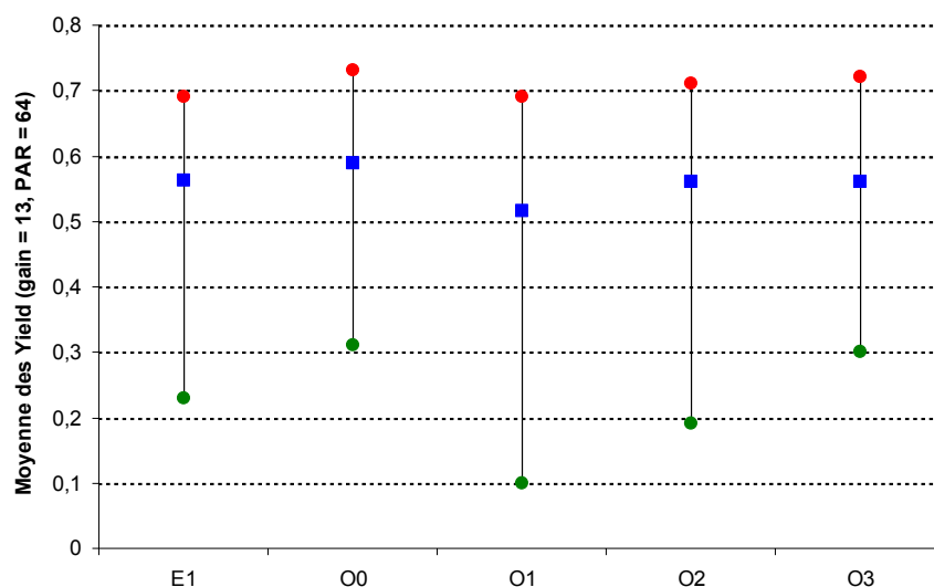
Figure 6 : Mesures de fluorimétrie sur les feuilles de lagarosiphon aux différentes stations
