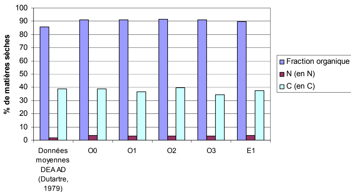
Figure 4 : Teneurs en matières organiques, azote et carbone des segments index des plantes dans les différentes stations (% des matières sèches)
