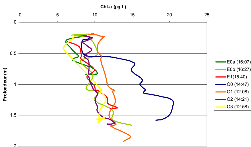
Figure 7 : Mesures des teneurs en pigments chlorophylliens des eaux dans les diverses stations de suivi à l'aide de la sonde fluoroprobe
