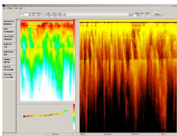
Figure 2 : Exemple de profils réalisés à l'échosondeur
