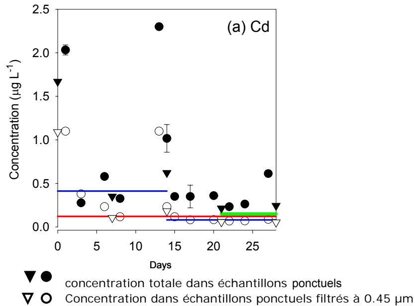
Figure 8 : Comparaison des concentrations moyennes en Cd par DGT pour des temps d'expositions de 7 (—), 14 (—) et 28 (—) jours avec les concentrations DGT totales mesurées sur des échantillons ponctuels bruts et filtrés de la Meuse (Mills et al., 2009).
