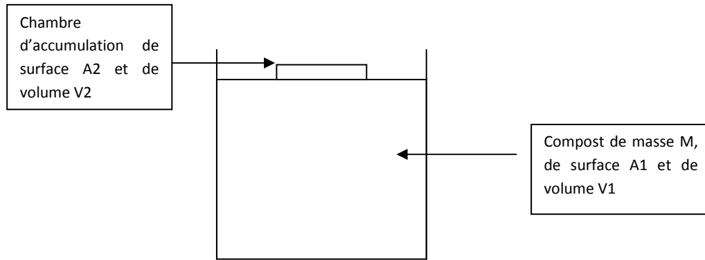
Figure 46 : Schéma de l'installation.
