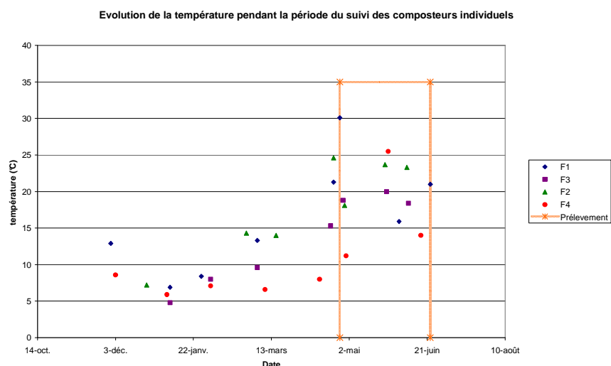
Figure 2 : Suivi de la température au sein des composteurs individuels.
