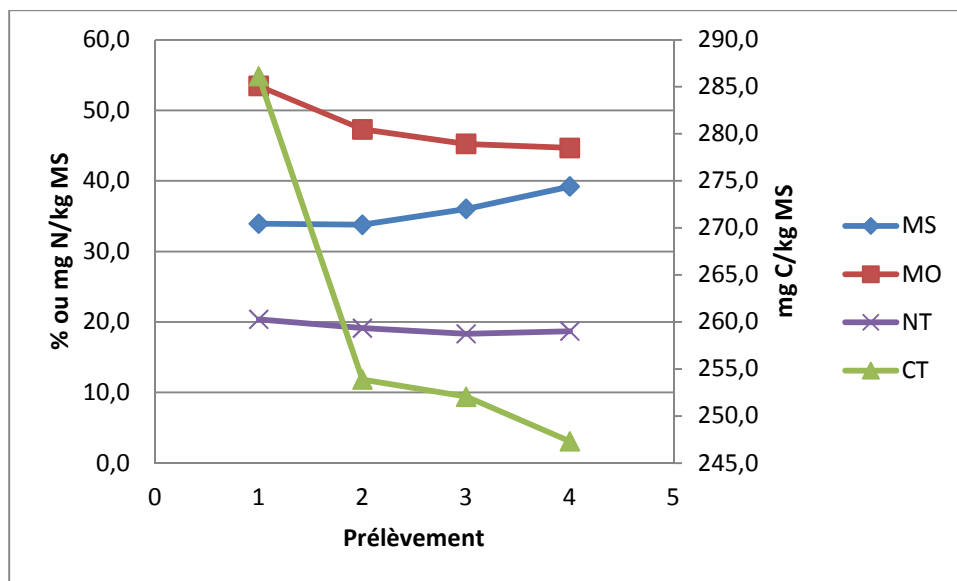
Figure 45 : Evolution des paramètres physico-chimiques au cours du compostage
