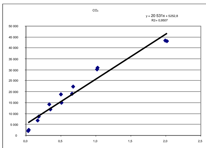
Figure 47 : Evolution de la concentration en CO 2 émis au cours du temps.
