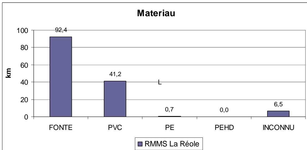
Figure 38 RMMS de La Réole Données matériau au niveau du service
