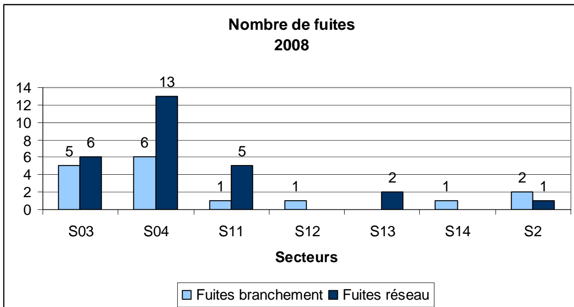
Figure 31 SIEA de Guîtres Nombre de fuites par secteur
