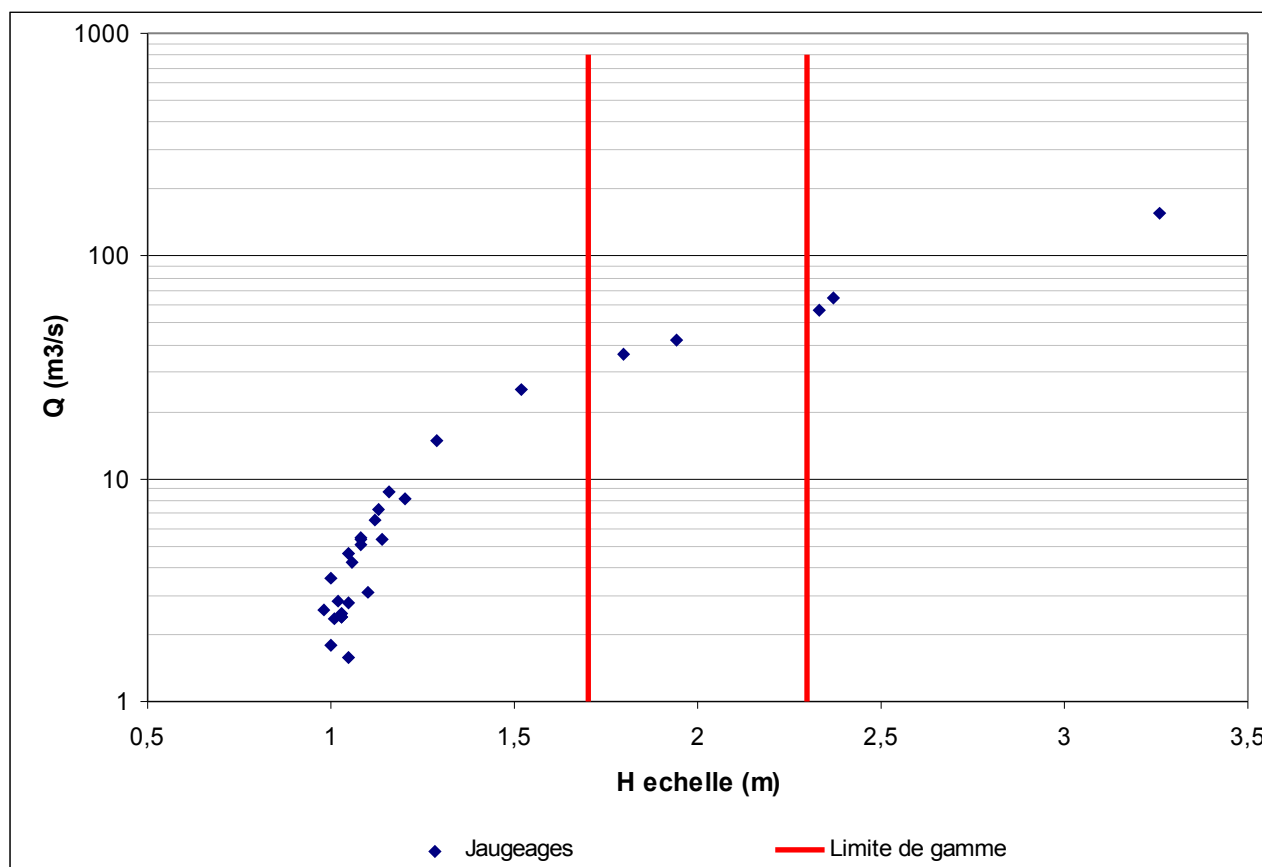
Figure 54: Jaugeages retenus pour l'analyse de la Sarre à Sarralbe Centre
