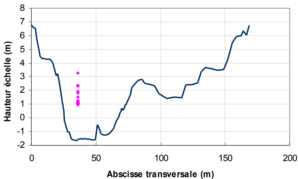
Figure 45: Section en travers du au droit du limnimètre de la station de Sarralbe centre sur la Sarre (en rose les hauteurs correspondant aux jaugages)
