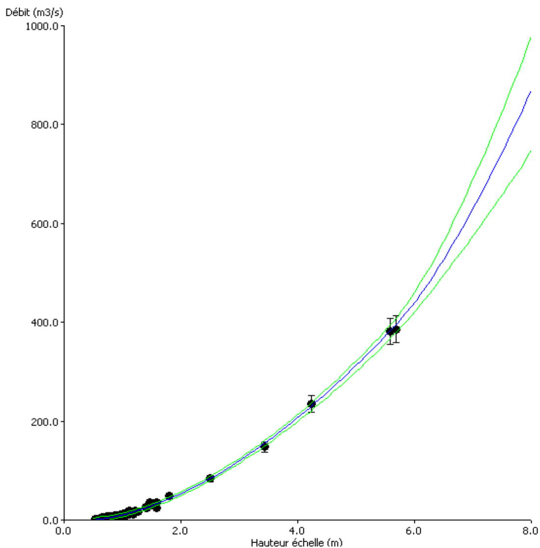
Figure 89: résultat graphique des courbes de tarage générées par BaRatin pour la station de Witting
