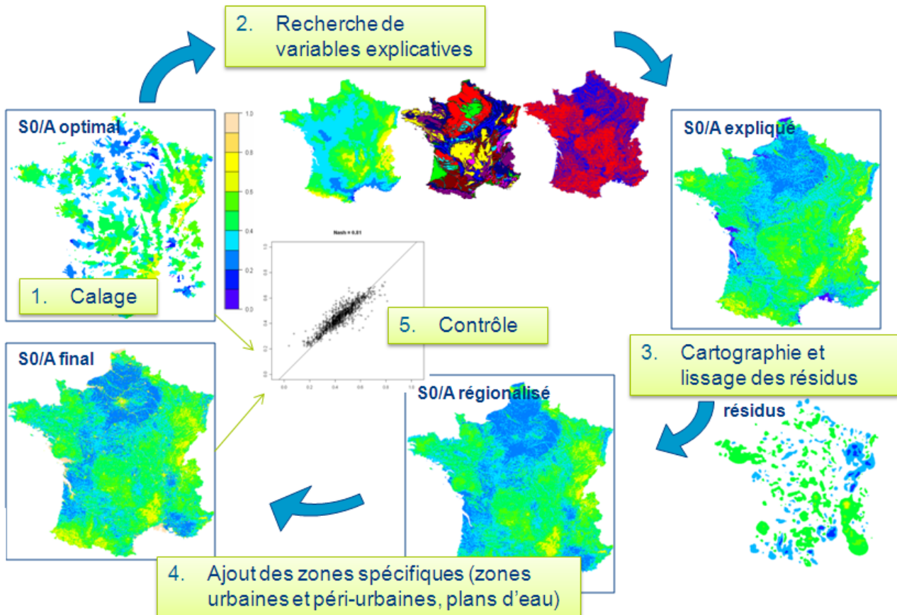
Figure 3 : Principe de la régionalisation du paramètre du modèle hydrologique.
