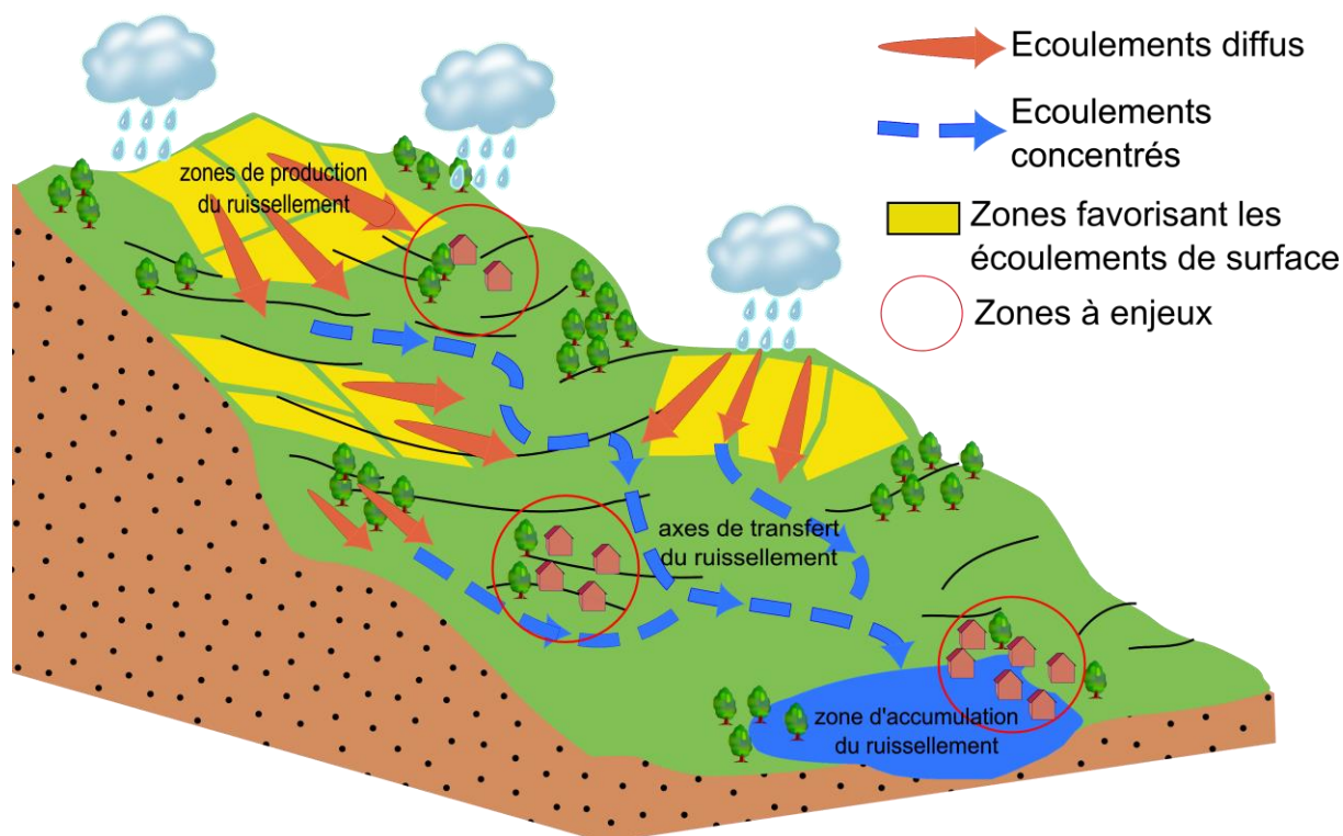
Figure 6 : Illustration des zones de production, de transfert et d'accumulation du ruissellement à l'échelle d'un bassin versant.
