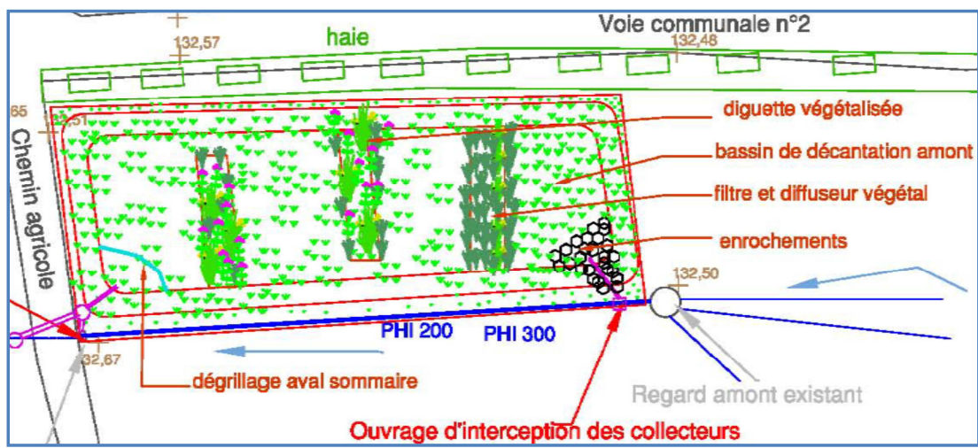
Plan d'une ZTHA avec insertion de diguettes
