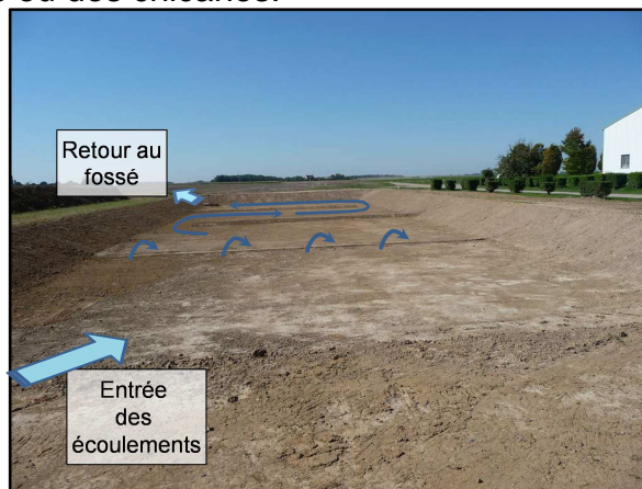
Bassin de Rampillon avec implantation de chicanes
