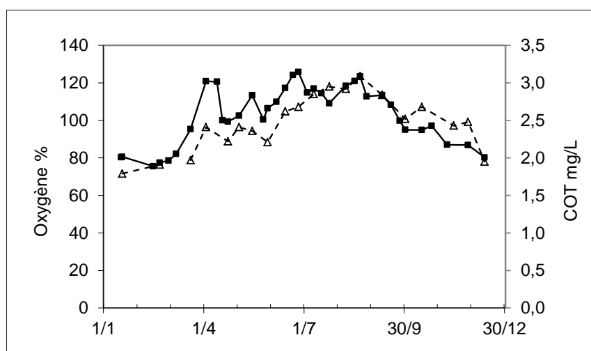
Figure 20 Evolutions saisonnières des concentrations en oxygène (—■—) (%) et en COT (- -△-) (mg.C.L -1 ) à 2 m de profondeur au point B en 2012
