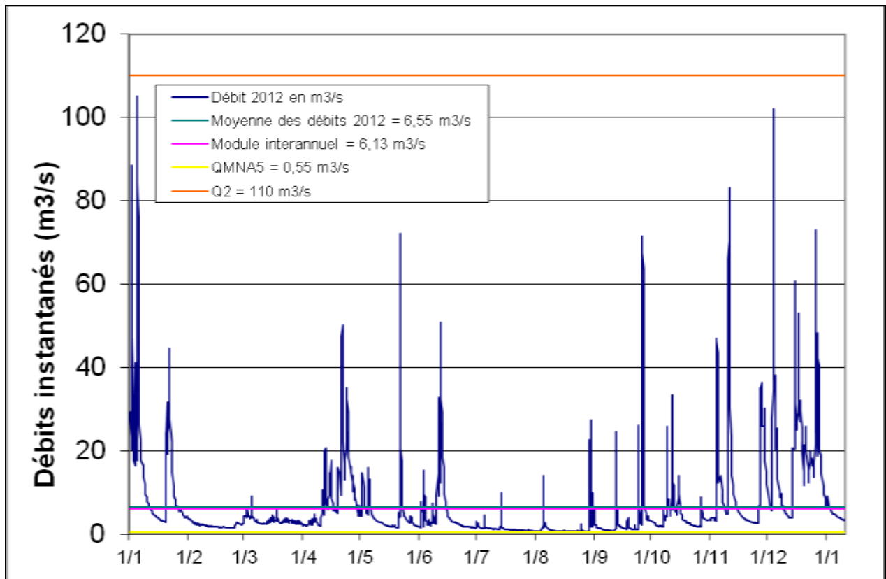
Figure 8 Chronologie des débits sur la Leysse en 2012 (source DREAL)
