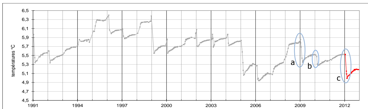
Figure 13 Températures à 140 m de profondeur au point B de 1991 à 2012
