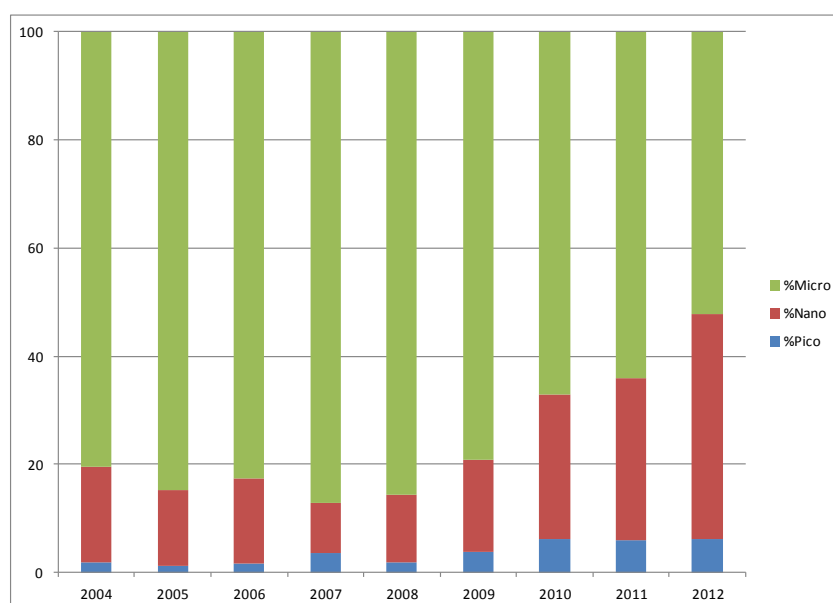
Fig 9 Evolution de la proportion en biomasse des compartiments pico-, nano- et microphytoplanctoniques dans le lac du Bourget depuis 2004
