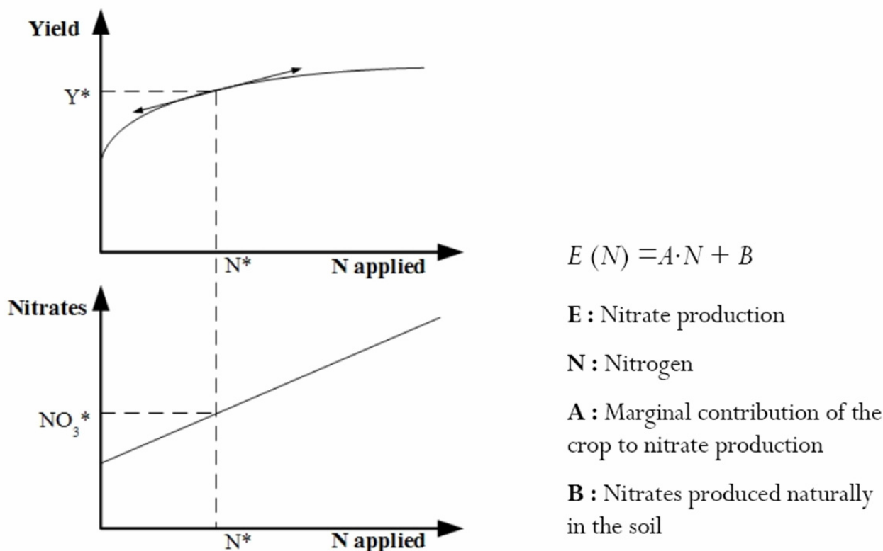
Figure 15 Fonction de réponse utilisée par AROPAj. La courbe du haut présente la relation entre le rendement et la dose d'azote utilisée (courbe obtenue d'après les simulations de Stics). AROPAj estime alors que le comportement optimal se situe là où la pente de la courbe est égale au rapport prix de l'azote/prix de vente de la culture. La dose d'azote ainsi estimée permet de déduire la quantité d'azote lixiviée (courbe du bas).
