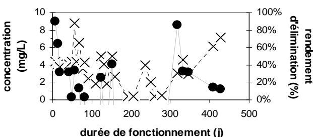
Figure 11 : Rendements d'élimination du COD, de l'ammonium et des phosphates par le filtre à charbon actif
