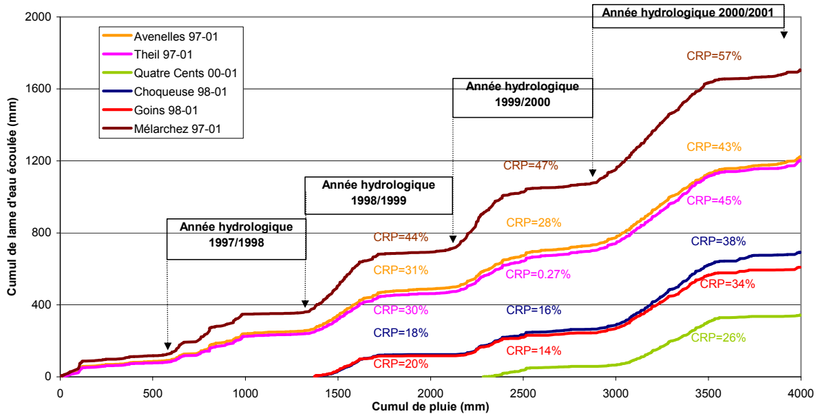
Figure 2: Représentation de la saisonnalité des écoulements des bassins d'ordre 1 à 3 du bassin versant de l'Orgeval
