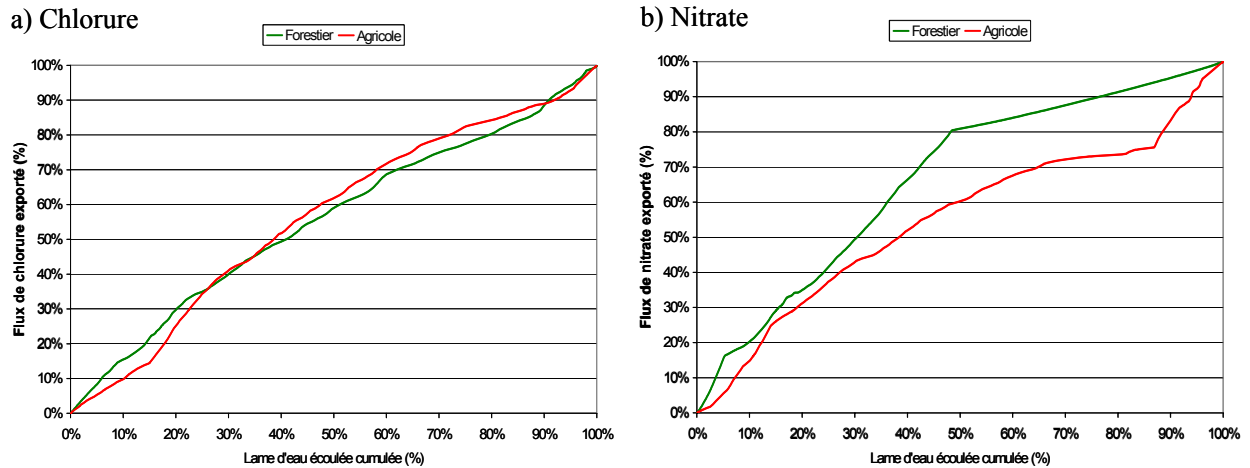
Figure 3: Dynamique temporelle des exportations de nutriments en fonction du cumul relatif de la lame d'eau écoulée sur les bassins forestier et agricole du 29/01/00 au 20/09/01, a) pour les Chlorures, b) pour les Nitrates
