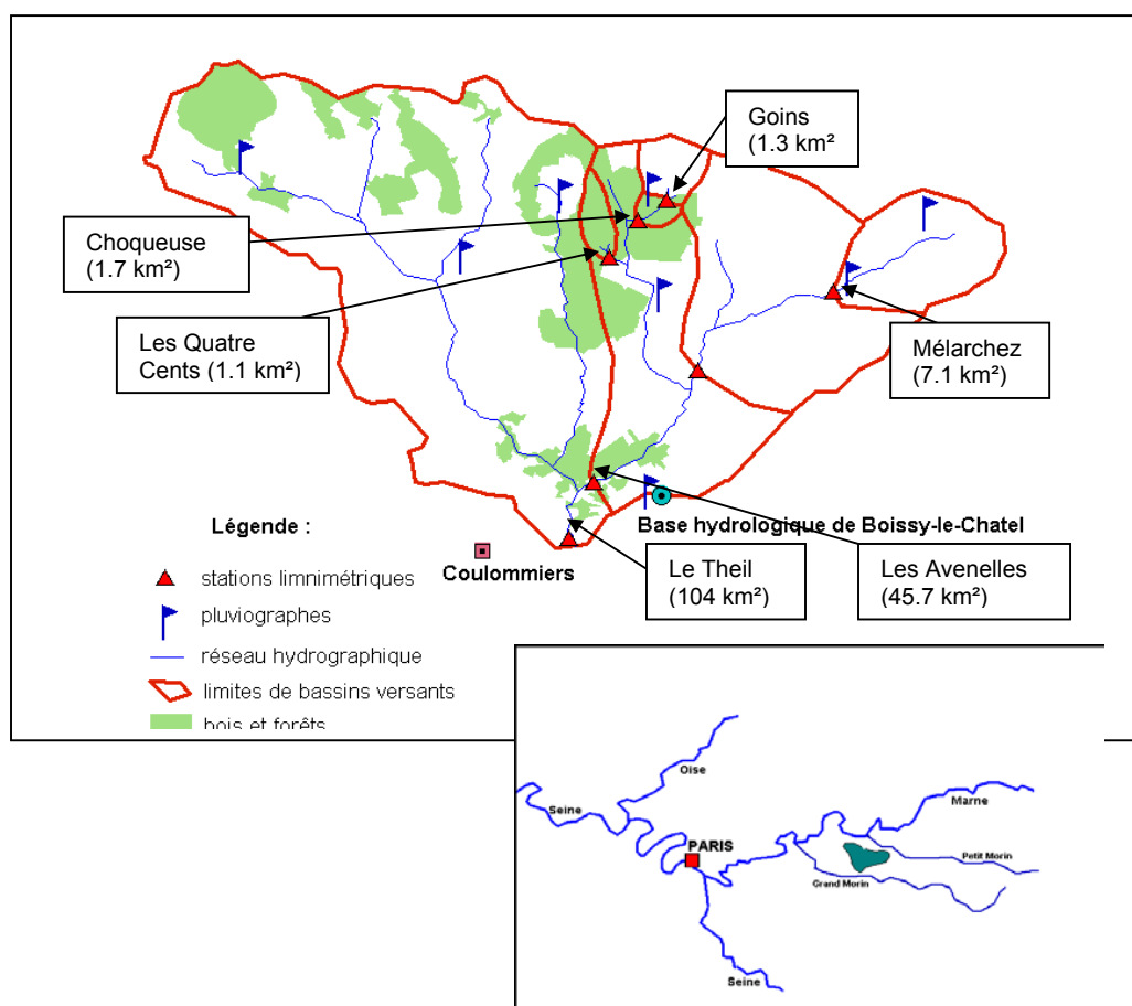
Figure 1: Localisation des sites étudiés sur le bassin versant de recherche de l'Orgeval.
