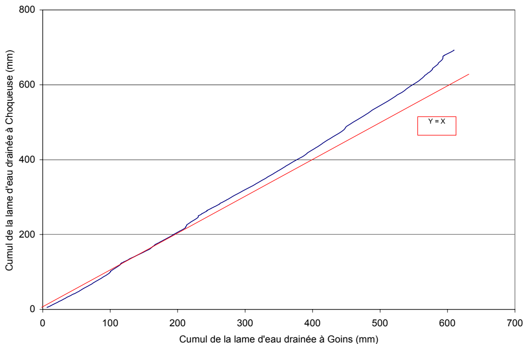
Figure 8 : Double cumuls des lames d'eau drainées à Goins et Choqueuse
