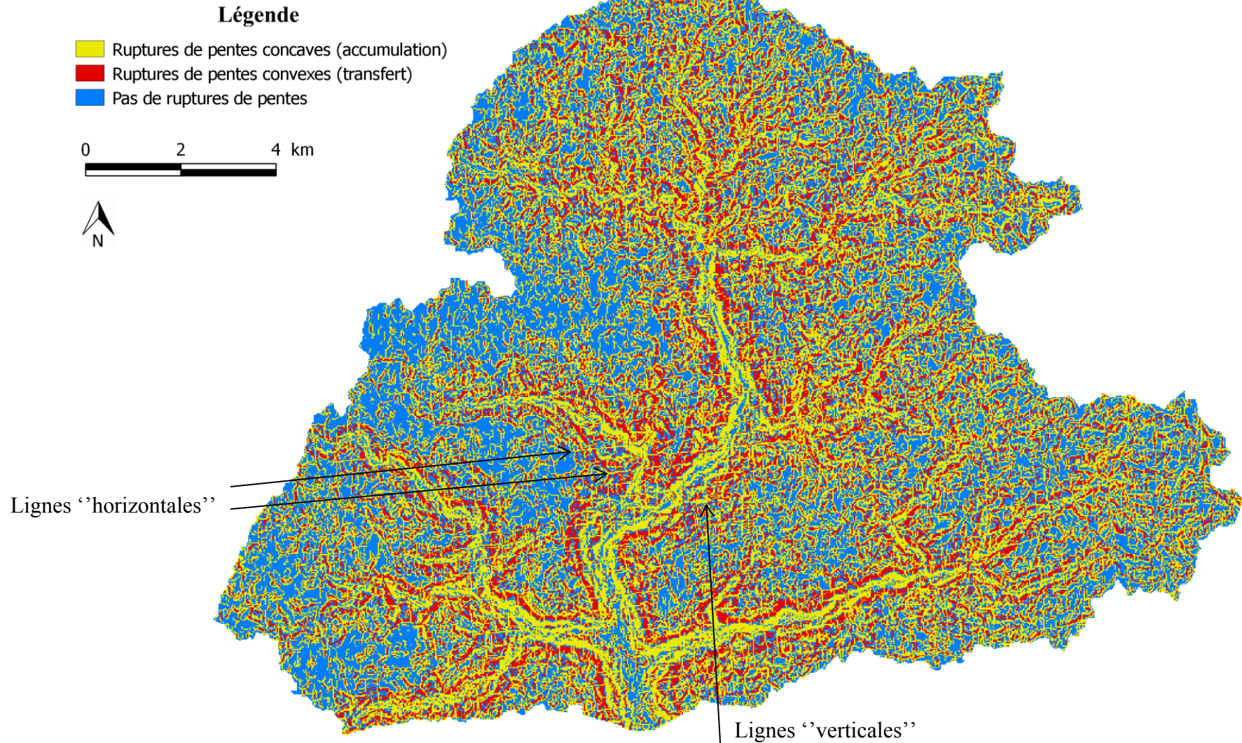
Carte synthétique des indicateurs de ruptures de pentes sur le bassin versant de la Lézarde Obtention sous iRIP
