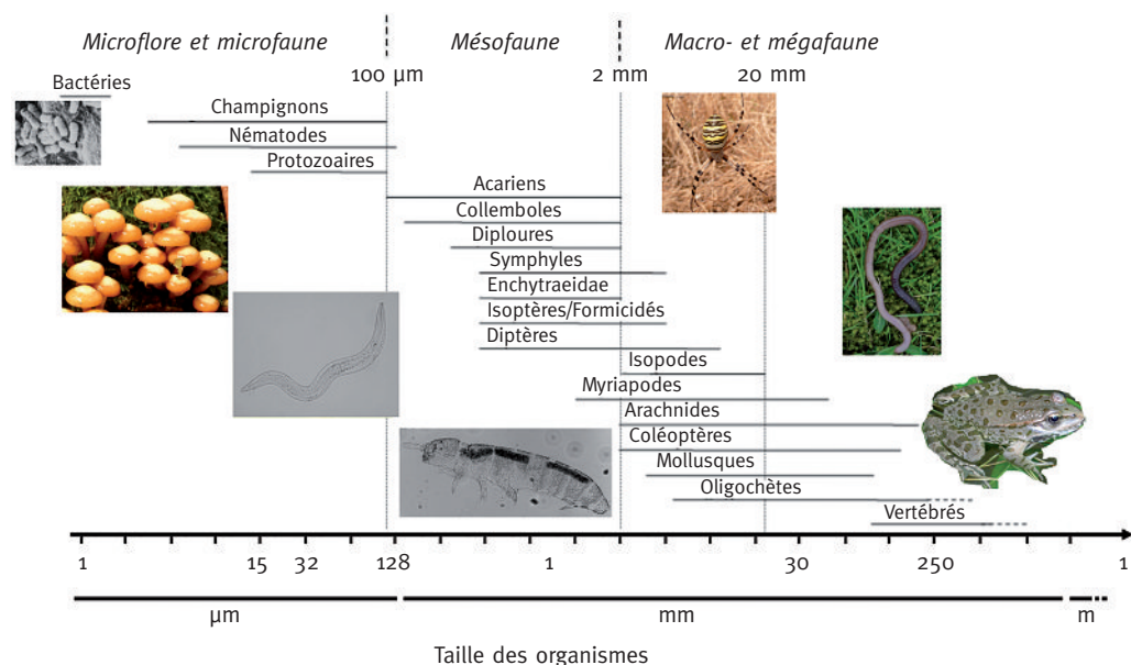
FIGURE 1 DISTRIBUTION DES ORGANISMES DU SOL EN FONCTION DE LEUR TAILLE (Adapté de T. Decaens, 2010)
