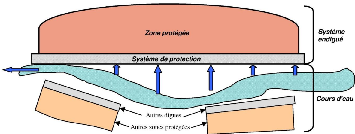
Figure 1.1 : Les trois composantes principales d'un système endigué fluvial : milieu(x) extérieur(s) « cours d'eau », système de protection et milieu extérieur « zone protégée » (d'après B. Beullac 2011)
