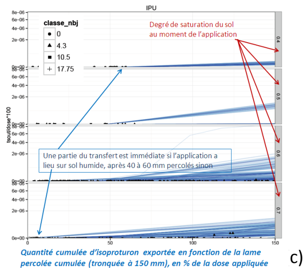
Figure 5 : dynamique d'exportation des substances actives, en fonction des lames d'eau écoulées.
