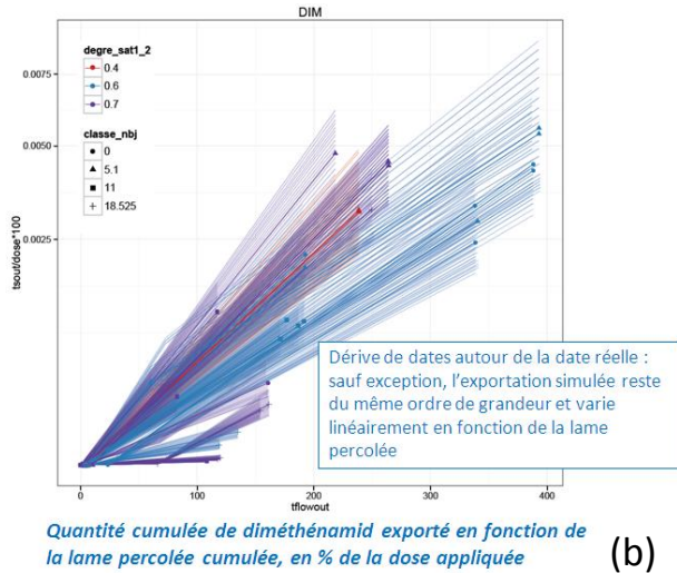
Figure 5 : dynamique d'exportation des substances actives, en fonction des lames d'eau écoulées.
