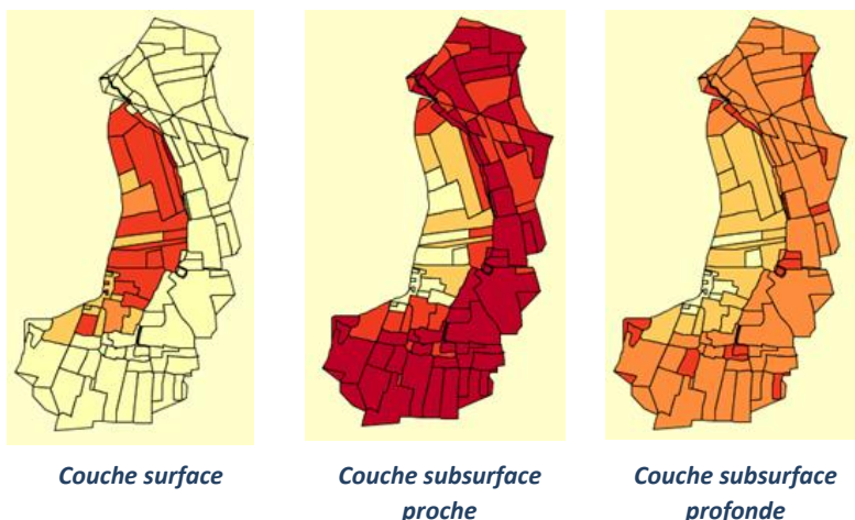
Figure 28 : Contribution des différentes couches de l'écoulement au transfert d'isoproturon. Période du 20 au 28 mars 2001. Simulation basée sur les résultats issus des parcelles T1 et T3 de la Jaillière
