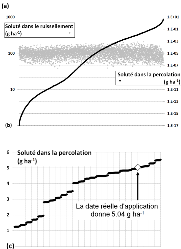
Figure 3 : Illustration de l'application « Cascade d'incertitudes ». Chaque point des vignettes b et c correspond à une simulation sur la période de 9 ans pour un jeu de paramètres
