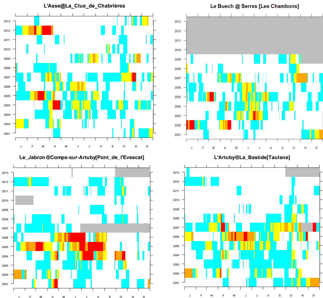
Figure 73 : Dispositif reposant sur le suivi des QC7 et seuils définis par les quantiles de VC3 décadaires (bleu : Vigilance ou Pré-alerte, jaune : Alerte, orange : Alerte renforcée, rouge : Crise, gris absence de données ; calculs réalisés sur toute la période disponible)
