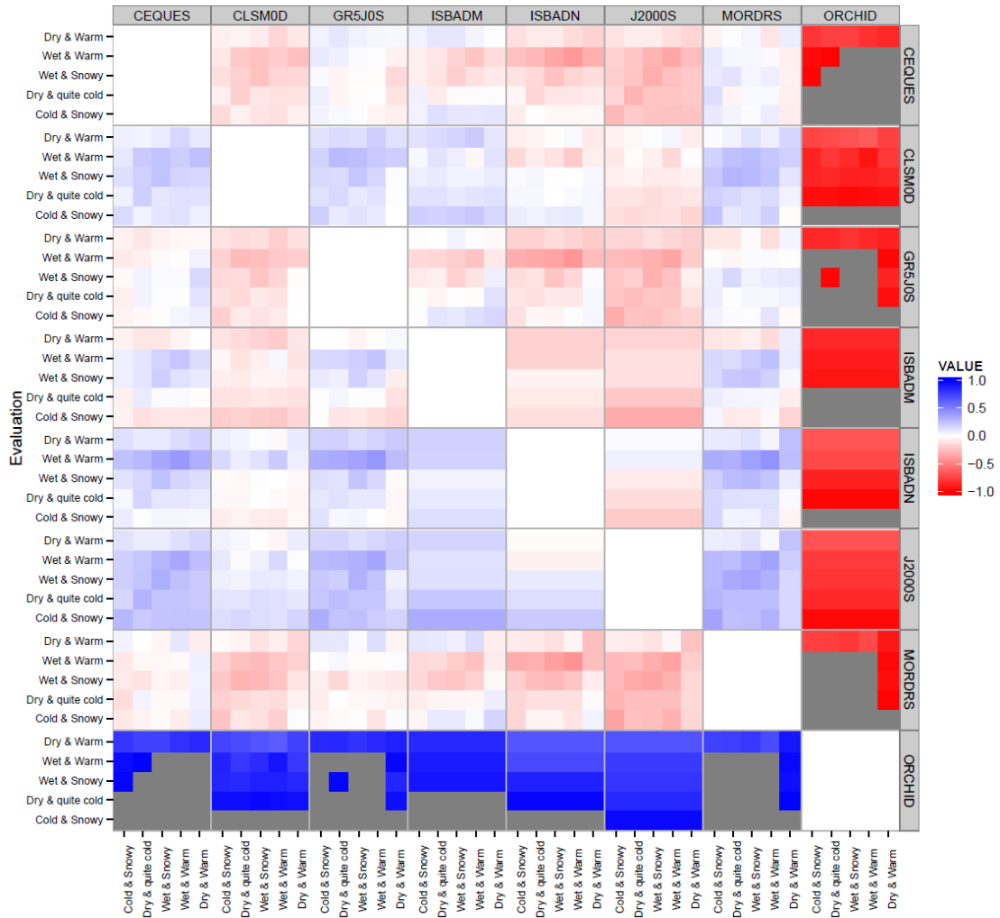
Figure 39 : Différences de performance en Nash-Sutcliffe sur les débits selon la période de calage et d'évaluation. Médiane de l'ensemble des stations. Une valeur positive, en bleu, indique que le modèle en colonne est plus performant que le modèle en ligne.
