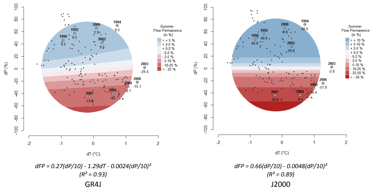
Figure 81 : Analyse de sensibilité du Flow Permanence estival, calculé du 15 avril au 15 octobre, fonction des anomalies climatiques sur la période juin-novembre (● scénario KNN ; ○ année observée)
