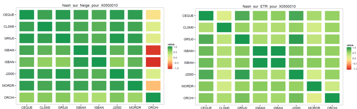
Figure 42 : Matrices de similarité pour la neige (gauche) et l'évapotranspiration réelle ETR (droite) de la Durance à Serre-Ponçon
