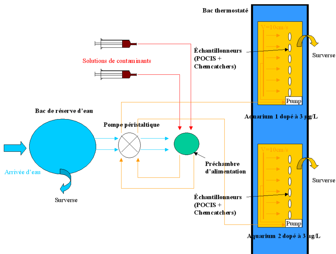
Figure 10. Schéma de fonctionnement du pilote utilisé par le participant MALY. Système ouvert avec un débit fixe pour chacun des 2 aquariums de 12,15 mL/min d'eau fraîchement dopée à environ 3 \mu\text{g/L} à l'aide des solutions de contaminants (préparées dans des solvants organiques). Le COD atteint environ 10 mg/L dans les aquariums (contre initialement < 1 mg/L dans l'eau de ville), ceci étant lié à l'introduction continue de solvants organiques (acétone, acétonitrile et méthanol) en même temps que les analytes d'intérêt. Les vitesses de courant dans les aquariums sont d'environ 10 cm/s au niveau de chaque POCIS) (Camilleri et al., 2012; Morin et al., 2013).
