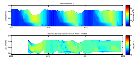
Figura 4: Temperatura estimada (arriba) y error (abajo) de la simulación con EOLE para el periodo de calibración.
