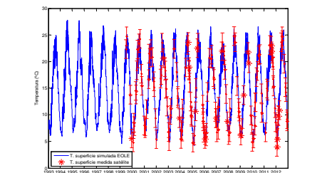
Figura 6: Comparación de la simulación con EOLE para 1999-2012 con las medidas de temperatura superficial por satélite.
