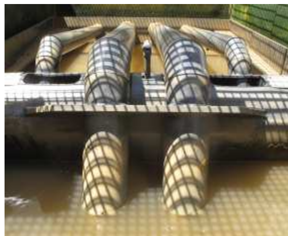
Siphon auto-amorçant du 1 er étage
