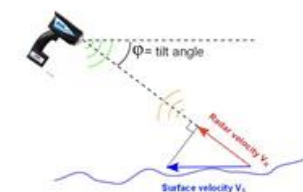
Principe de fonctionnement du radar vélocimétrique
