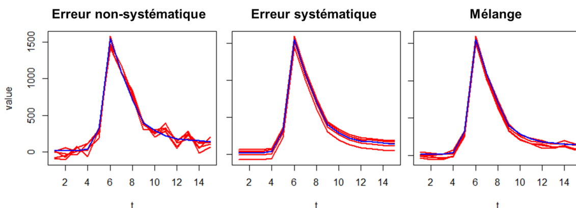
Figure 7-17 : Illustration de la différence entre des spaghettis issus d'erreurs non-systématiques (à gauche), purement systématiques (au milieu) ou d'un mélange d'erreurs systématiques et non-systématiques (à droite). Noter que si l'incertitude était représentée sous forme d'intervalles et non de spaghettis, on obtiendrait exactement les mêmes intervalles dans les trois cas.
