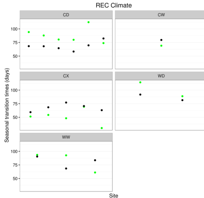
Figure 7-15 : Temps de transition saisonnier moyen (été-hiver : noir ; hiver-été : vert) pour les stations de mesure d'humidité des sols regroupées par classe climatique d'après la classification REC (Snelder et al., 2005) : CD : cool dry ; CW : cool wet ; CX : cool extremely wet ; WD : warm dry ; WW : warm wet.
